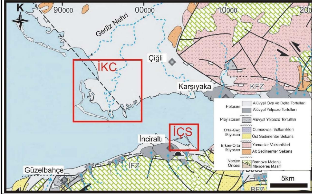
Şekil 1. Yer bulduru ve jeoloji haritası [38].
