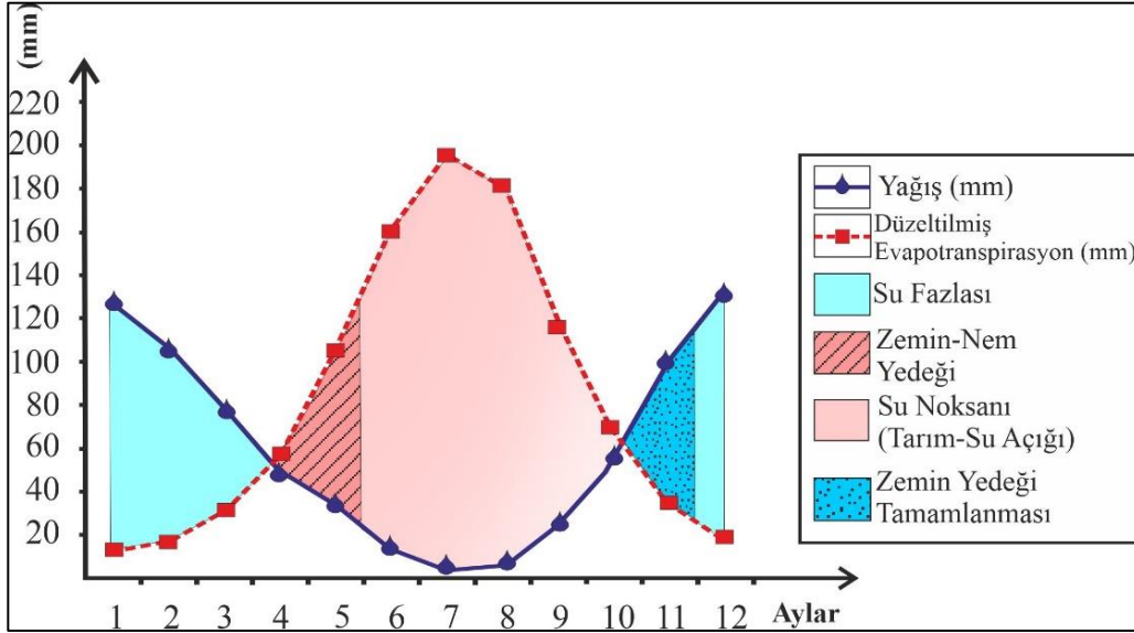
Şekil 2. İzmir ili Thorntwaite Grafiği.
