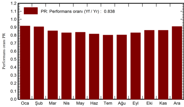
Şekil 3.3 7° Kuzey yönü Polikristal panelli sistemin yıllık ortalama performans oranı (Figure 3.3. Average annual performance rate of system with north facing 7° orientation angle Polycrystalline panel)
