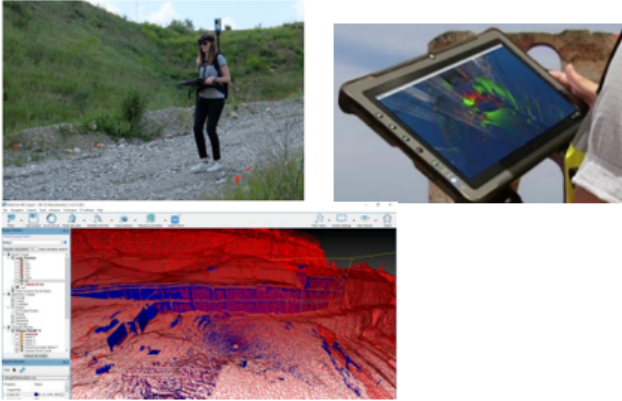
Şekil 18. Açık madende GML kontrol ünitesi ve 3B görüntüsü (Vassena ve Clerici, 2018).
