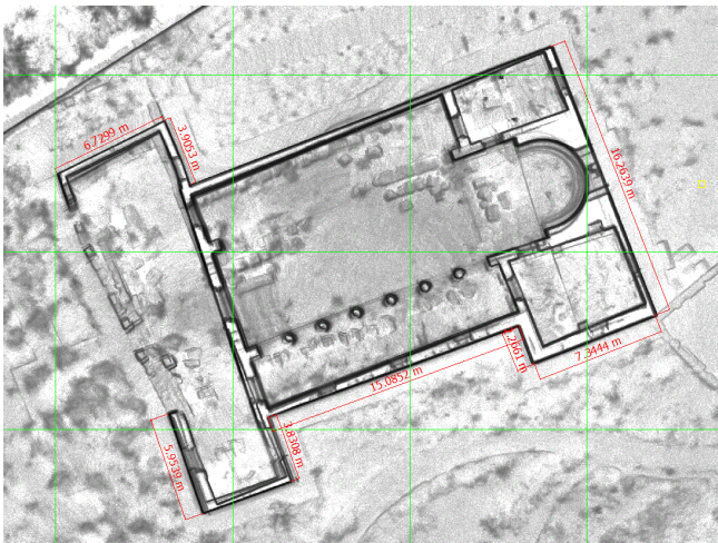
Şekil 37. Cambazlı kilisesinin ortofotosu üzerinden ölçülen uzunluklar.
