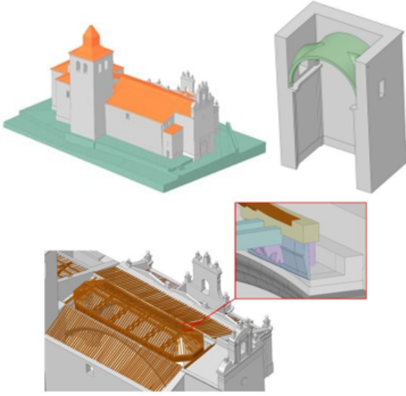
Şekil 11. Adanero Kilisesi'nin 3B modelleri ayrıntıları çizimde gözükmektedir (Rodríguez, 2022).
