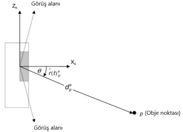
Şekil 1. Lazer taramada iki boyutlu plan görünümü (Barber vd., 2008).
