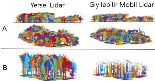
Şekil 12. A ve B arazilerindeki orman ağaçlarının giyilebilir mobil tarayıcı ve Yersel Lidar ile rastgele renklendirilmiş 3B modeli (Coba, vd., 2018).
