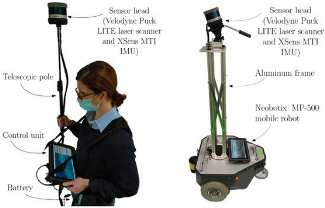
Şekil 17. GML tarayıcının elle ve platform üzerinde taşınması (Maset, vd., 2022).
