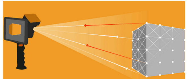
Şekil 4. Mobil LİDAR ile taranmış bir tünelin 3B nokta bulutu (Geoslam 2021).
