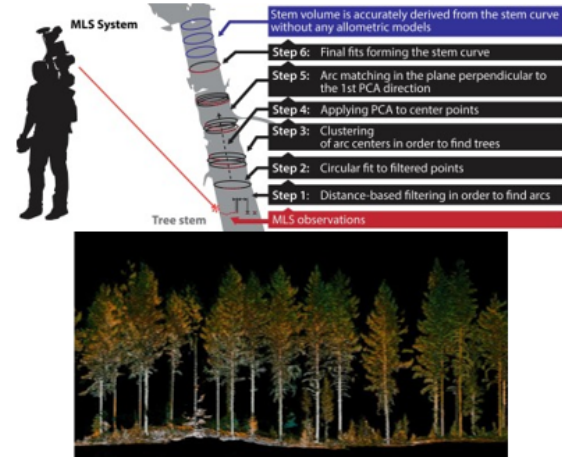
Şekil 13. Orman ağaçlarının giyilebilir mobil tarayıcıyla ölçümü ve 3B modeli (Hyypä, vd., 2020).
