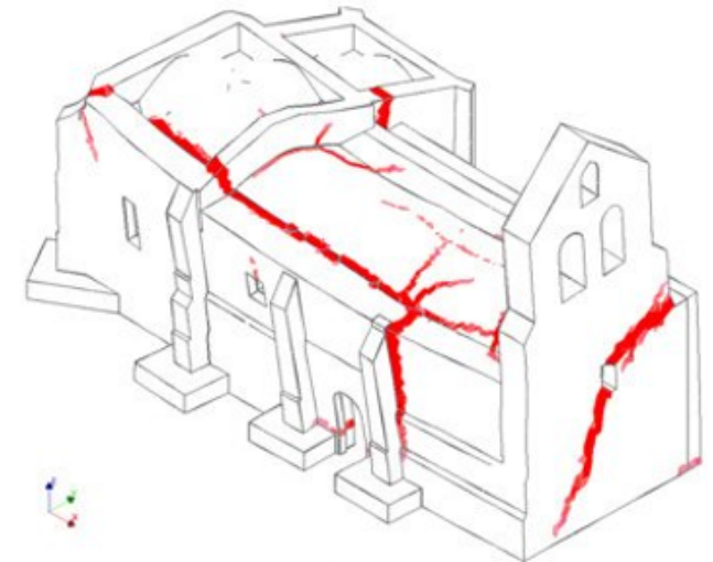
Şekil 19. San Pedro Kilisesi'nin birinci şekilde kapalı tarama güzergâhı ikinci şekilde -y yönündeki çökmesi gözükmektedir (Sánchez-Aparicio vd. 2021).
