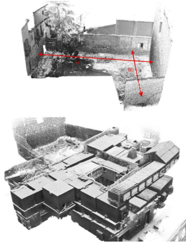
Şekil 10. Birinci şekil doğruluk değerlendirmesi için ölçülen mesafeler, ikinci şekil nokta bulutunu göstermektedir (Filippo, 2018).
