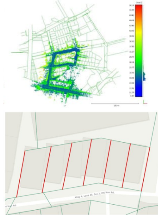
Şekil 22. Giyilebilir Lidar ile birinci şekil filtreleme sonunda nokta bulutu, ikinci şekil muhtemel kadastro sınırlarının çizimi (Chio ve Hou, 2021).
