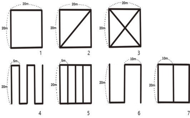
Şekil 14. Sırt çantasındaki mobil lazer tarama cihazı ile ormandaki taramalar için kullanılan farklı alım yolları (Ko, vd., 2021).
