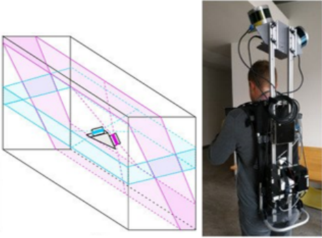
Şekil 23. Araştırmada tespit edilen en iyi çift Lidar konumu (Velas, vd., 2019).
