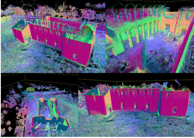
Şekil 35. Cambazlı kilisesinin farklı açılardan 3B modeli
