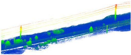
Şekil 24. ENH hattı 3B model (Velas, vd., 2019).
