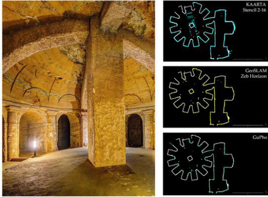
Şekil 21. Mağaranın resmi ve farklı markalı mobil tarayıcılarla on iki gen kubbenin plan kesiti (Di Stefano, vd., 2021).
