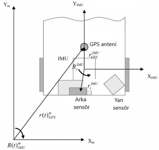
Şekil 2. GPS anteni, IMU ve lazer profil oluşturucu plan görünümü (Barber vd., 2008).
