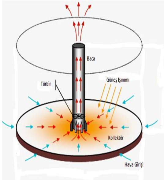
Şekil 1 Güneş bacası sisteminin çalışma prensibi [7]
