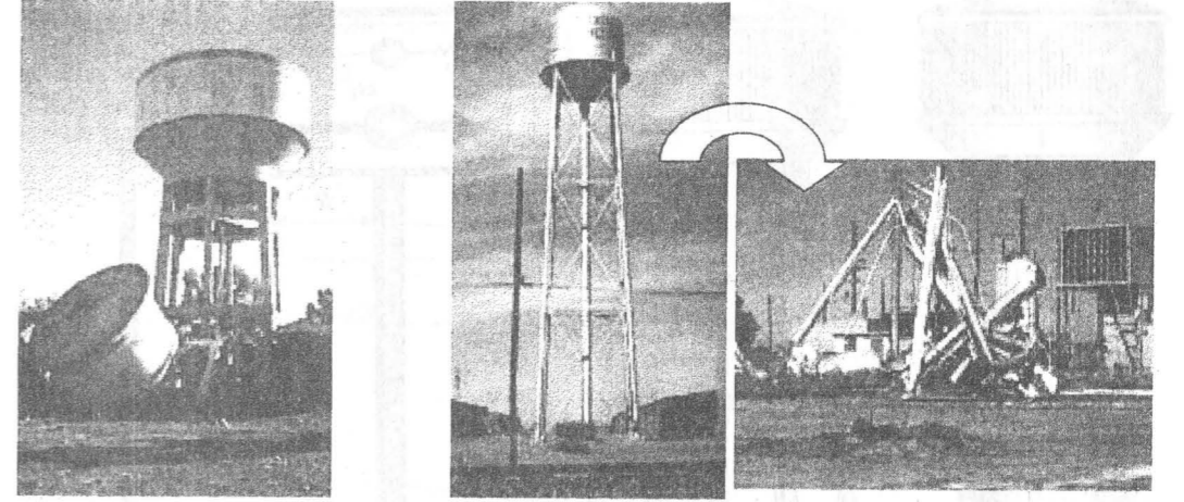
Şekil 1. Depremlerde yıkılmış betonarme ve çelik ayaklı depo görüntüleri
