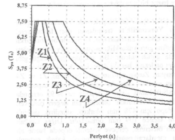
Şekil 4. Çalışmaya konu depolar için alınacak ivme spektrumları
