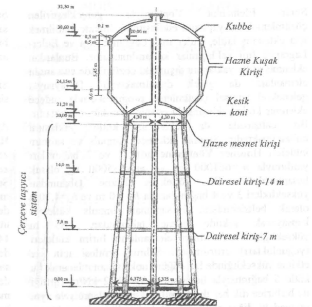
Şekil 5. Çerçeve taşıyıcı sisteme sahip deponun düşey kesiti
