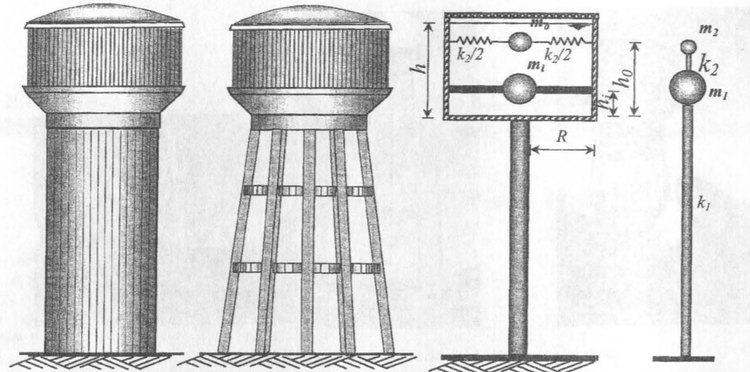
Kabuk taşıyıcı sisteme sahip ayaklı depo Çerçeve taşıyıcı sisteme sahip ayaklı depo Eşdeğer mekanik Model Matematik Model Şekil 2. Ayaklı depoların mekanik eşdeğeri ile matematik modeli
