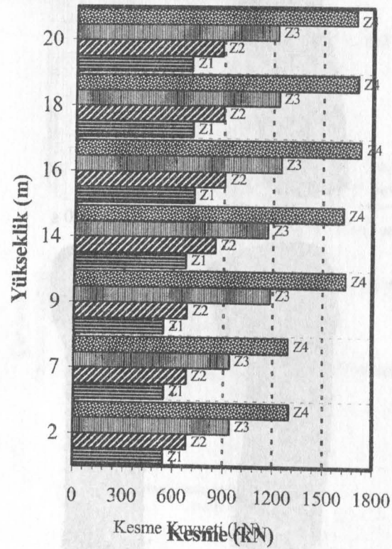
Şekil 10. Çerçeve sistemli deponun düşey taşıyıcı elemanlarındaki, farklı zemin koşulları için maksimum kesme kuvveti değişimi.
