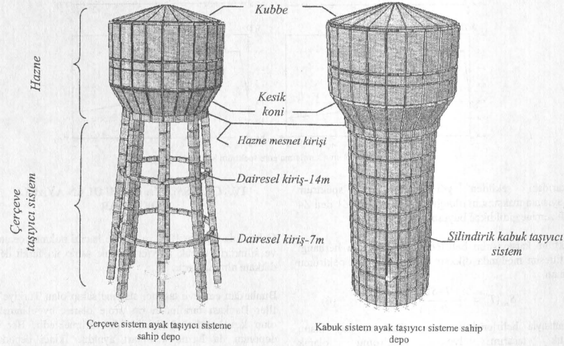
Şekil 6. Seçilen depoların sonlu eleman modelleri
