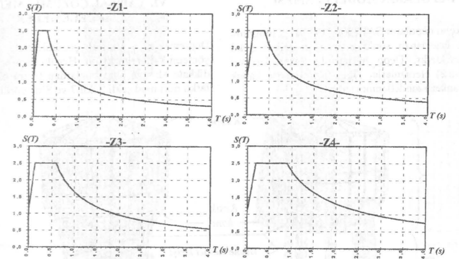
Şekil 3. Zemin sınıflarına göre spektrum katsayısının değişimi
