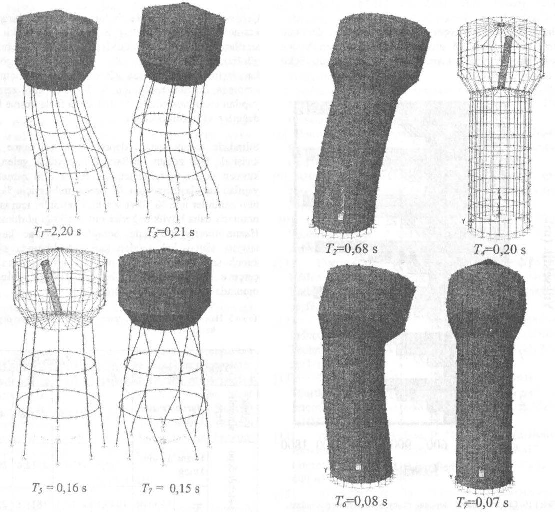
Şekil 7. Çerçeve sistemli ayaklı deponun 4 farklı mod şekli ve periyotları
