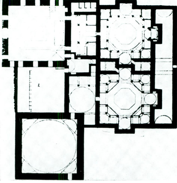
Res. 13 — Cağaloğlu Hamamı plânı (H. Glück)
