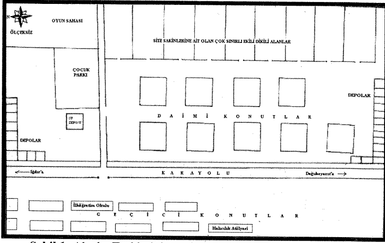
Şekil 1. Ahıska Türklerinin yerleştirildiği sitenin plânı.
