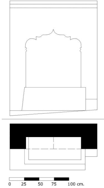
Çizim-3: Çeşmenin plan ve cephe görünüşü Foto.4: Çeşmenin genel görünüşü (Çizim-Lokman Tay)
