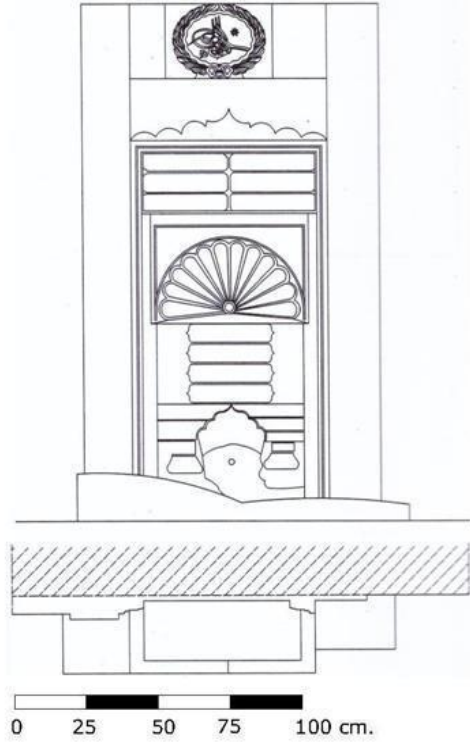
Çizim-1: Çeşmenin plan ve cephe görünüşü Foto.1: Çeşmenin genel görünüşü (Koçyiğit, 2013: 111-115)
