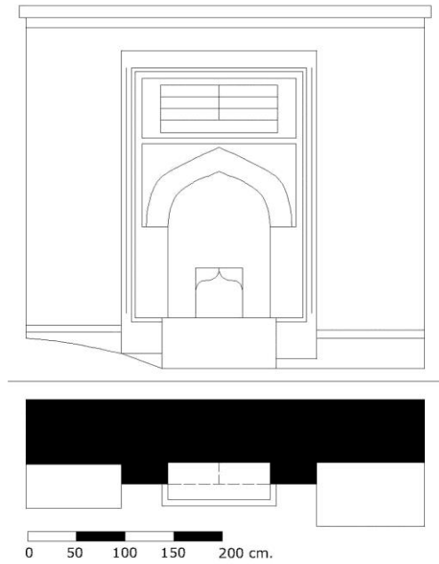
Çizim-6: Eyüp Hacı Beşir Ağa Çeşmesi plan ve cephe görünüşü (Çizim-Lokman Tay)
