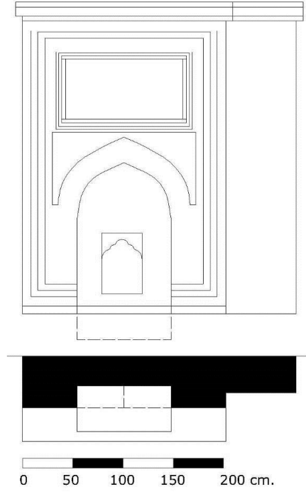
Çizim-5: Çeşmenin plan ve cephe görünüşü (Çizim-Lokman Tay)
