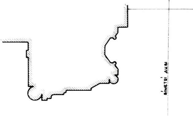
CAMİ PORTALI-KESİT
