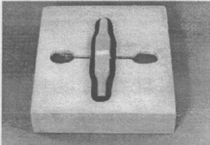
Resim 1. PMMA bloklar arasında yumuşak astar maddesinin polimerize edildiği sert alçı düzenek.
