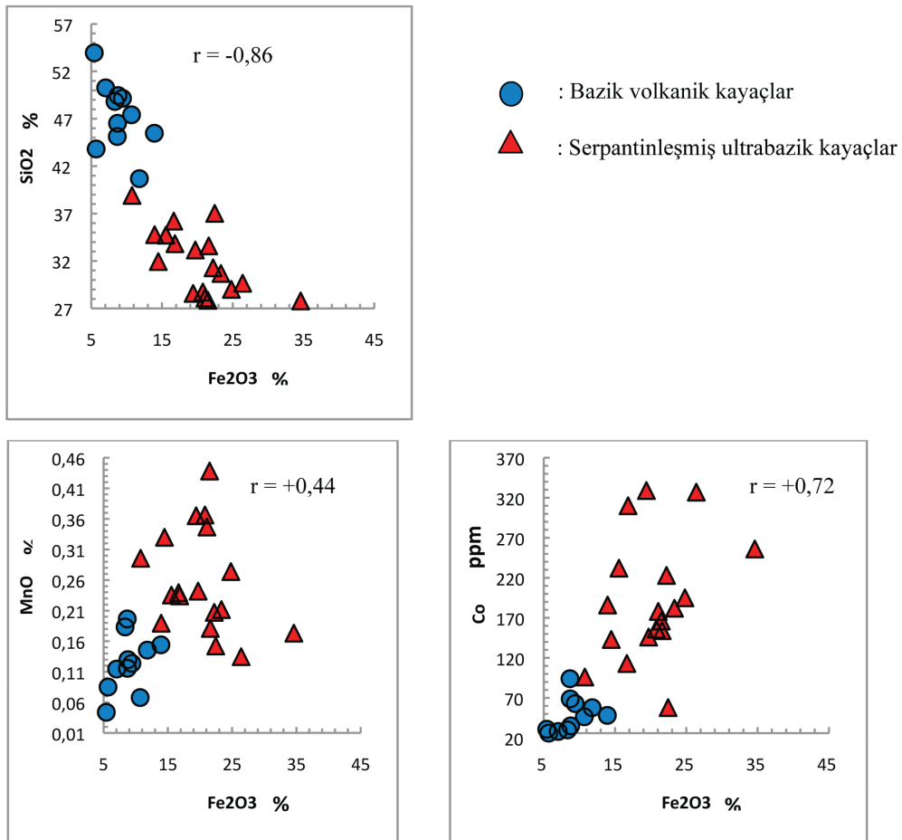
Şekil 21. Tüm kayaç örneklerinde (serpantinleşmiş ultrabazik kayalar + bazik volkanik kayalar; toplam 29 örnek) toplam \text{Fe}_2\text{O}_3 'e karşı; \text{SiO}_2 , MnO ve Co element dağılım grafikleri ( r = korelasyon katsayısı değeri).
