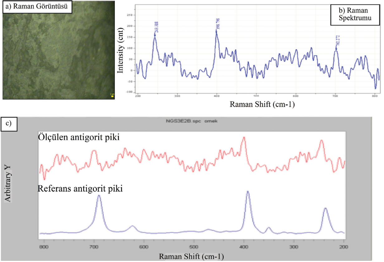
Şekil 12. Y-86 örneğine özgü Raman spektroskopisi verileri.
