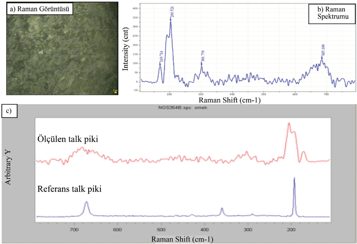
Şekil 11. Y-79 örneğine özgü Raman spektroskopisi verileri.
