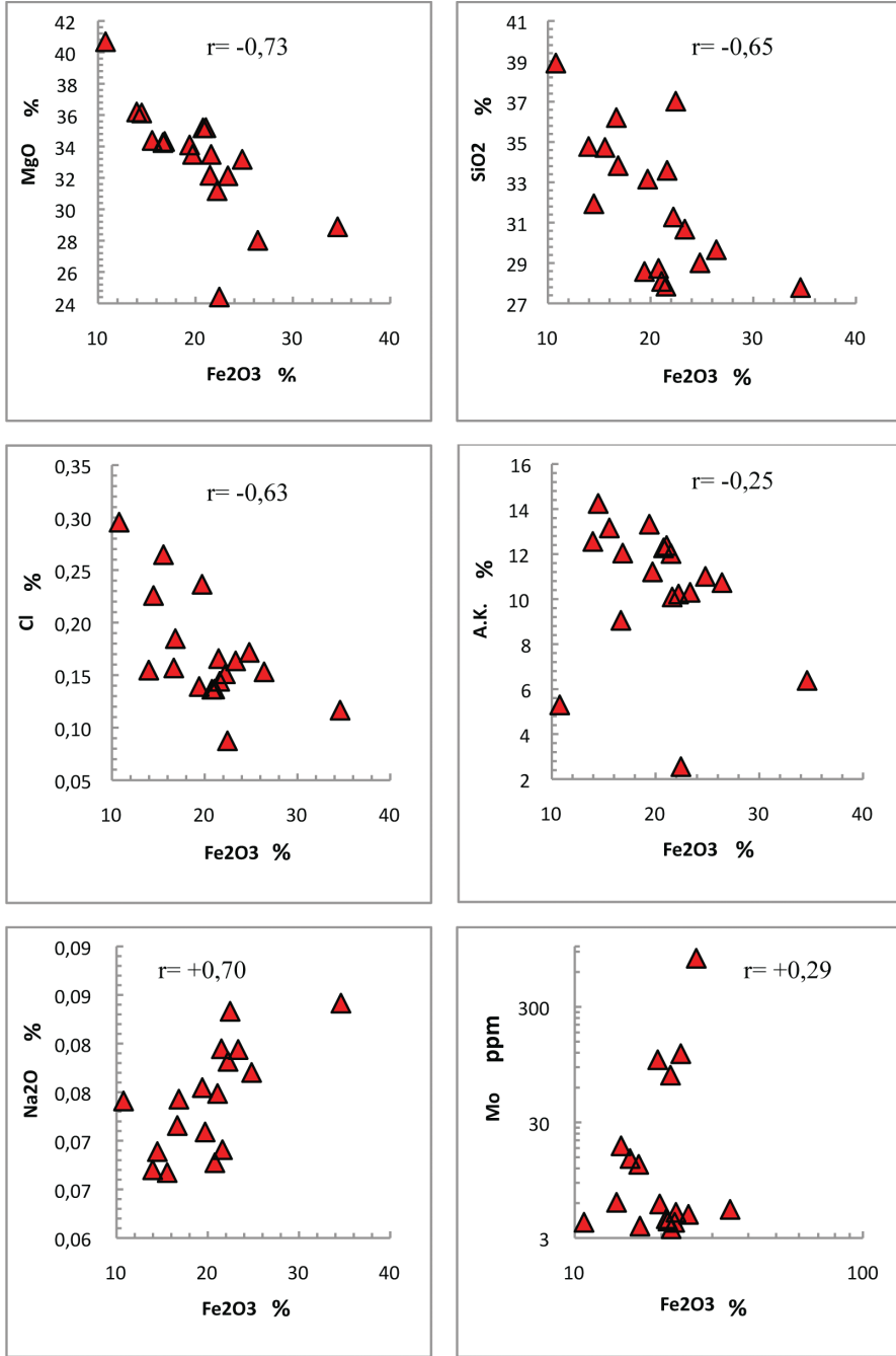
Şekil 22. Serpantinleşmiş ultrabazik kayaç örneklerinde (toplam 18 örnek) toplam Fe 2 O 3 'e karşı; MgO, SiO 2 , Cl, Na 2 O, Mo element ve A.K. dağılım grafikleri (toplam Fe 2 O 3 'e karşı Mo element dağılım grafiği log-log dağılımı olarak verilmiştir) ( r = korelasyon katsayısı değeri).
