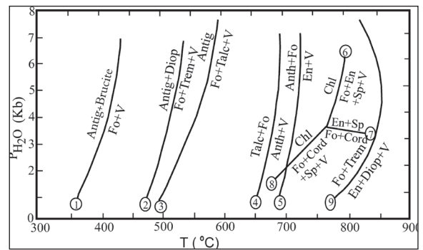
Şekil 25. Ultramafik metamorfik kayaçların yorumlanmasında kullanılan Mg-Si-Ca-O-H sistemindeki reaksiyonları gösteren PH 2 O -T diyagramı, Antig: Antigorit, Fo: Forsterit, V: Su/Buhar, Diop: Diyopsit, Trem: Tremolit, En: Enstatit, Chl: Klorit, Cord: Kordiyerit, Sp: Serpantin (Dymek vd., 1988).
