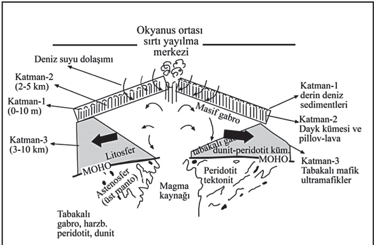
Şekil 23. Okyanus sırtlarında okyanus kabuğunun oluşumunun kesiti (Guilbert ve Park, 1986).
