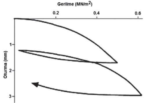
Şekil 4. Tipik bir gerilme - oturma - boşaltma grafiği.
