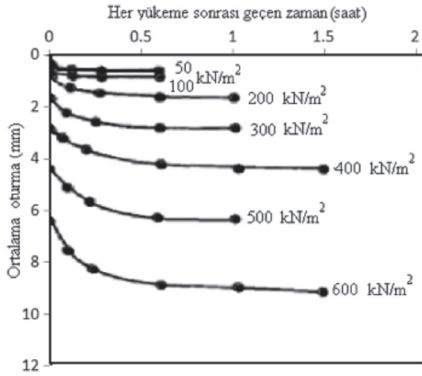
Şekil 3. Sabit yük kademeleri altında zamana bağlı oturma grafiği (Clayton vd.,1995).
