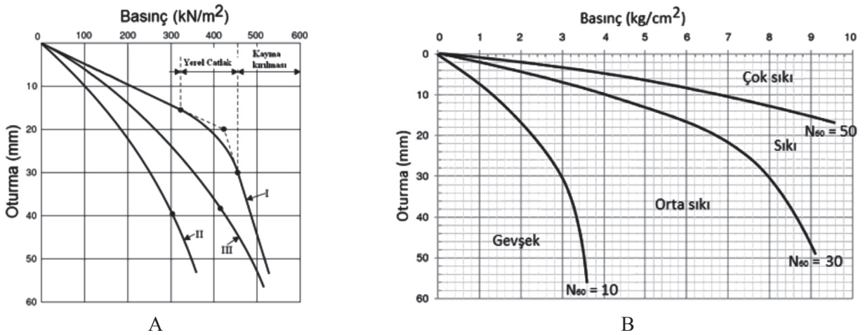
Şekil 5. A) Farklı zemin grupları için basınç - oturma eğrileri (Venkatramaiah, 1993), B) Kumlarda plaka yükleme deneyi eğrisi ile zemin sıklığı arasındaki ilişki (Terzaghi ve Peck, 1948).
