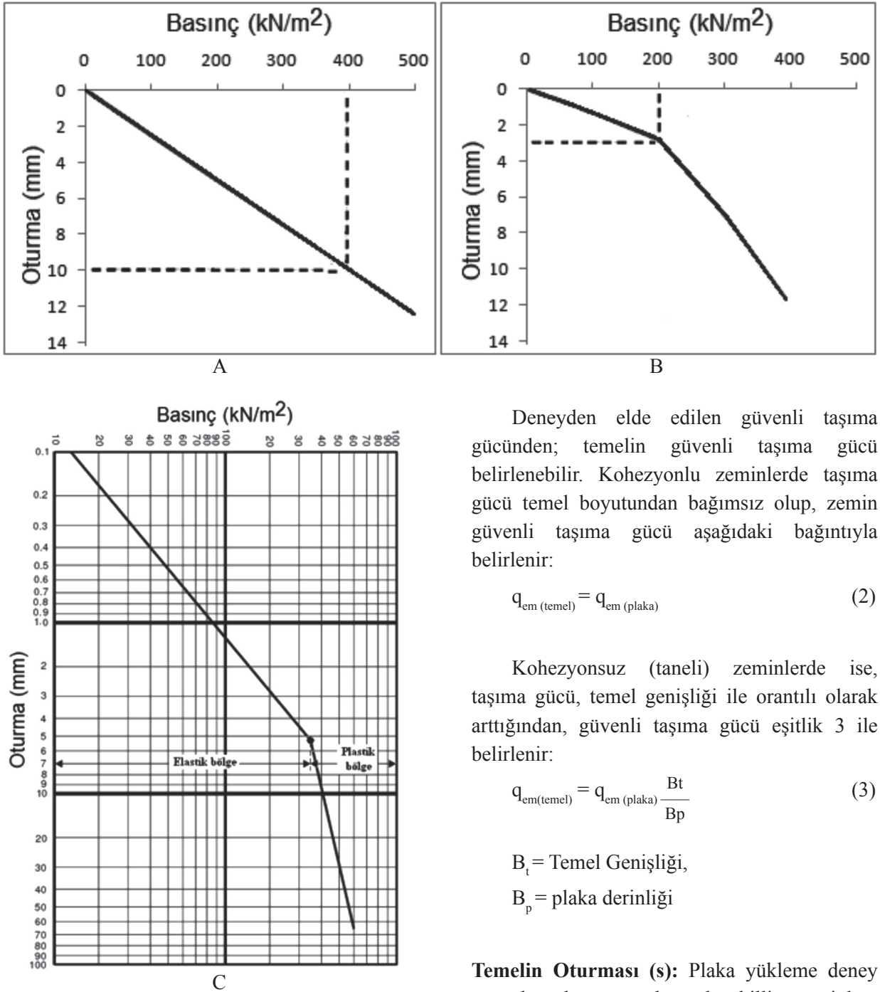
Şekil 6. Basınç – oturma grafiğinden taşıma gücünün belirlenmesi.
