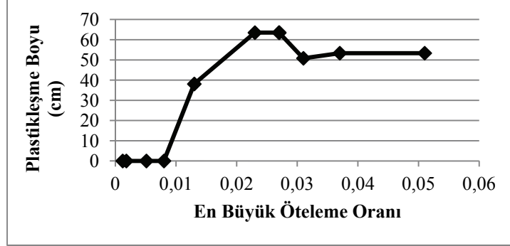
Şekil 4. Plastikleşme boyu
