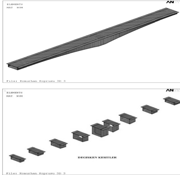
Şekil 12. Köprü boyunca değişken kesitler, sonlu eleman ağları
