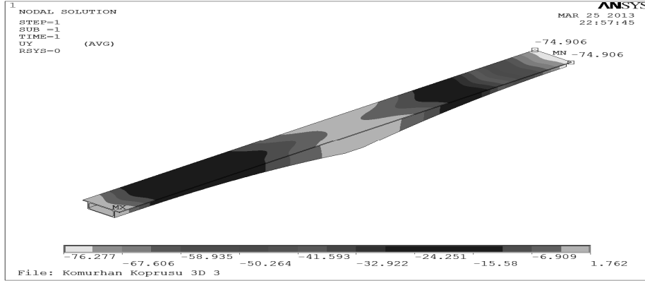
Şekil 22. Ek ölü yükler, kendi ağırlığı, H_{30}S_{24} kamyonları, yaya yükünden konsol ucunda oluşan düşey yerdeğiřtirme -74.9mm
