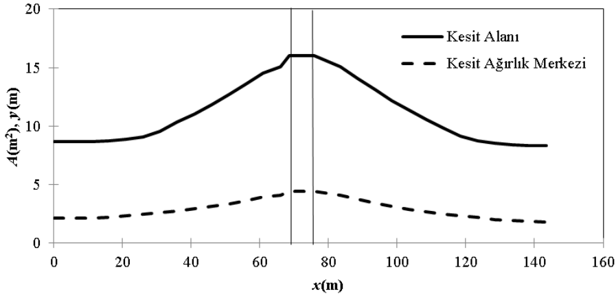
Şekil 6. Köprü boyunca değişken kesit alanı A ( m^2 ), kesit ağırlık merkezi y ( m )
