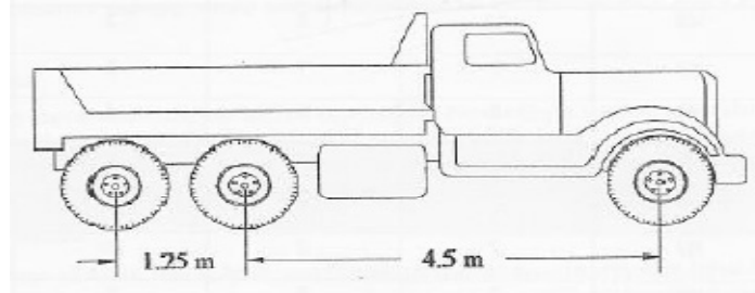
Şekil 15. Saha incelemesinde kullanılan kamyon
