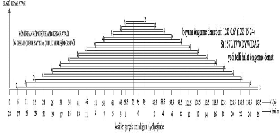
Şekil 11. Kesitlere göre boyuna öngerme donatı demeti sayısı
