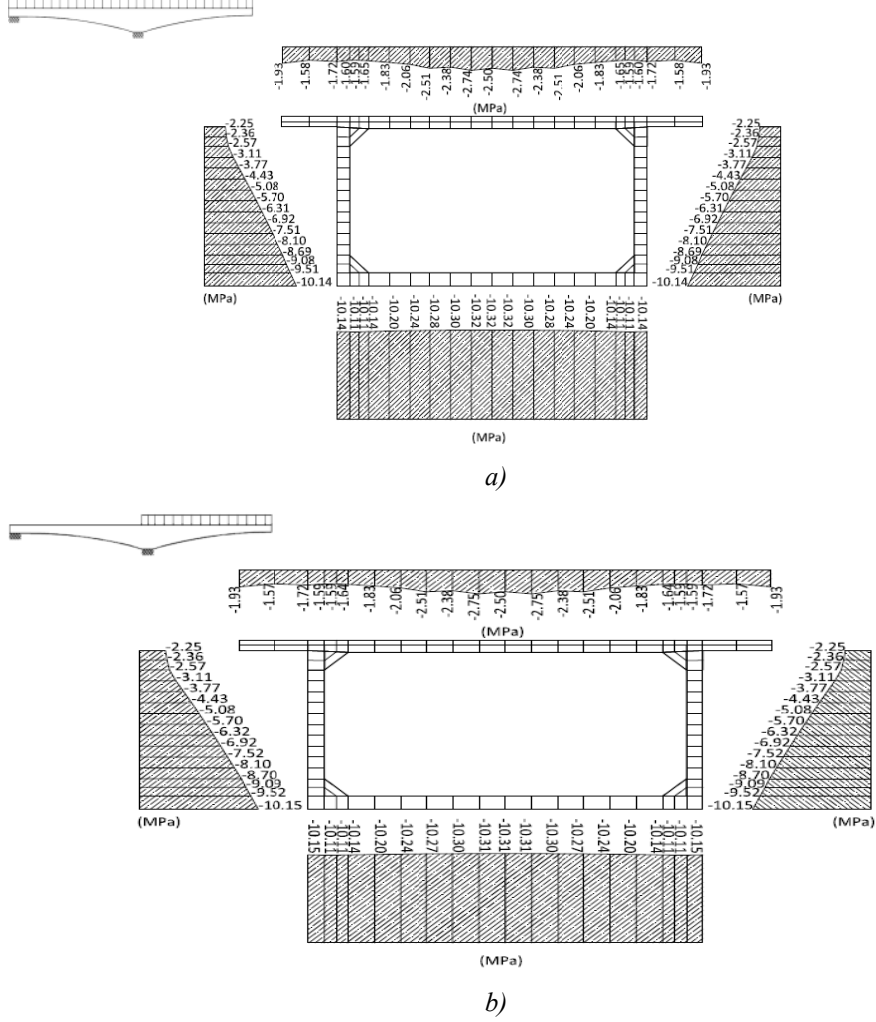
Şekil 27. Köprü ana ayak yüzünden x=9.2 m kadar uzakta normal gerilmeler, trafik yükü a) Köprü'nün bütününde, b) Yalnız ana açıklık konsolunda etkili
