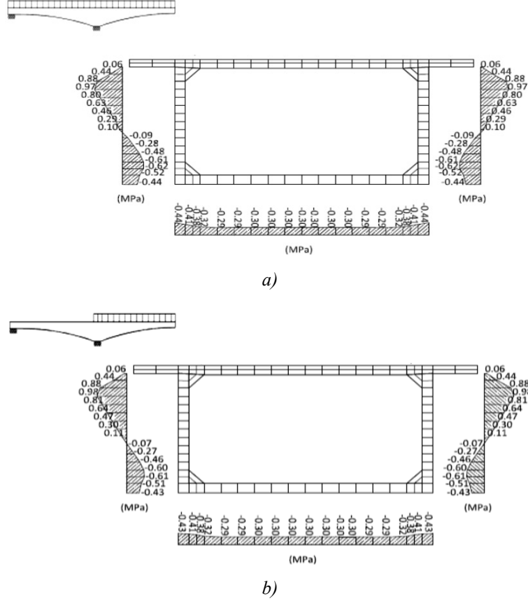
Şekil 28. Köprü ana ayak yüzünden x=9.2 m kadar uzakta kesme gerilmeleri, trafik yükü a) Köprü'nün bütününde, b) Yalnız ana açıklık konsolunda etkili
