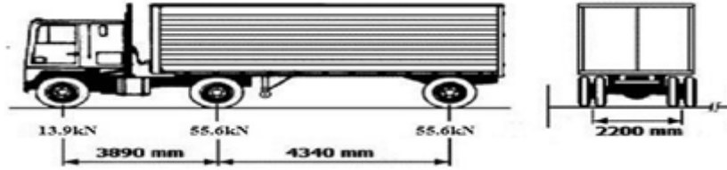
Şekil 8. En elverişsiz yükleme durumu için H_{30}S_{24} kamyonu
