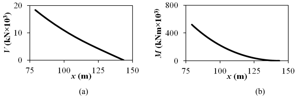
Şekil 9. Kendi ağırlığı, ek ölü yüklerden oluşan a) Kesme kuvveti, b) Eğilme momenti diyagramı
