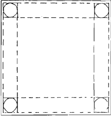
Çizim 9: Rukiye Dudu Türbesi Planı, Kesiti ve Görünüşü (Uveys'den)
