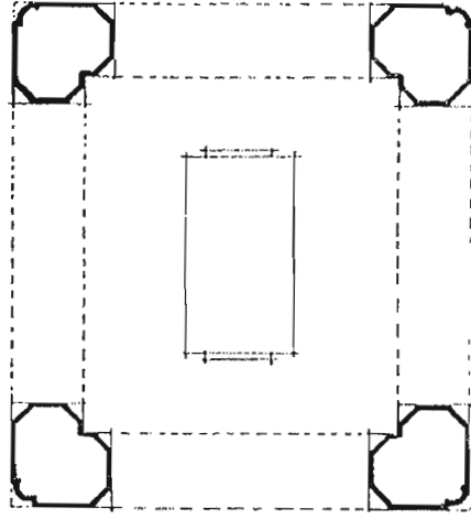
Çizim 1: Emir Burham Türbesi Planı (Badr'den).
