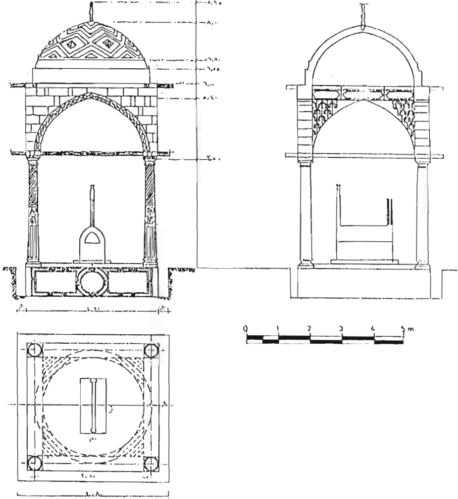
Çizim 6: Emine Kadın Türbesi Planı, Kesiti ve Görünüşü (Uveys'den)
