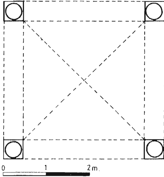
Çizim 8: Mustafa Bey Şahin Türbesi Planı
