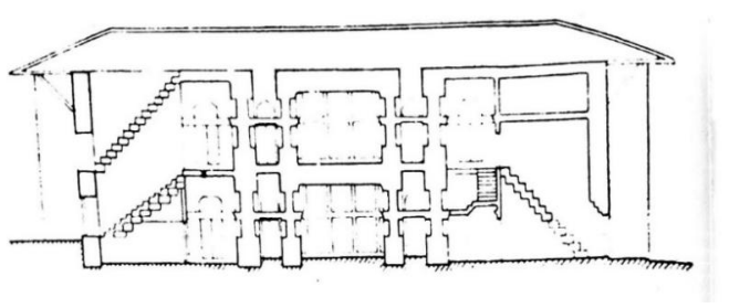
Çizim 1: Şeki Han Sarayının kesiti 2
