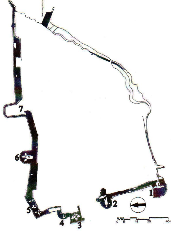
Çizim-1 Ayas (Yumurtalık) Kıyı Kalesi Planı (Boaz'dan Düzenlenerek).
