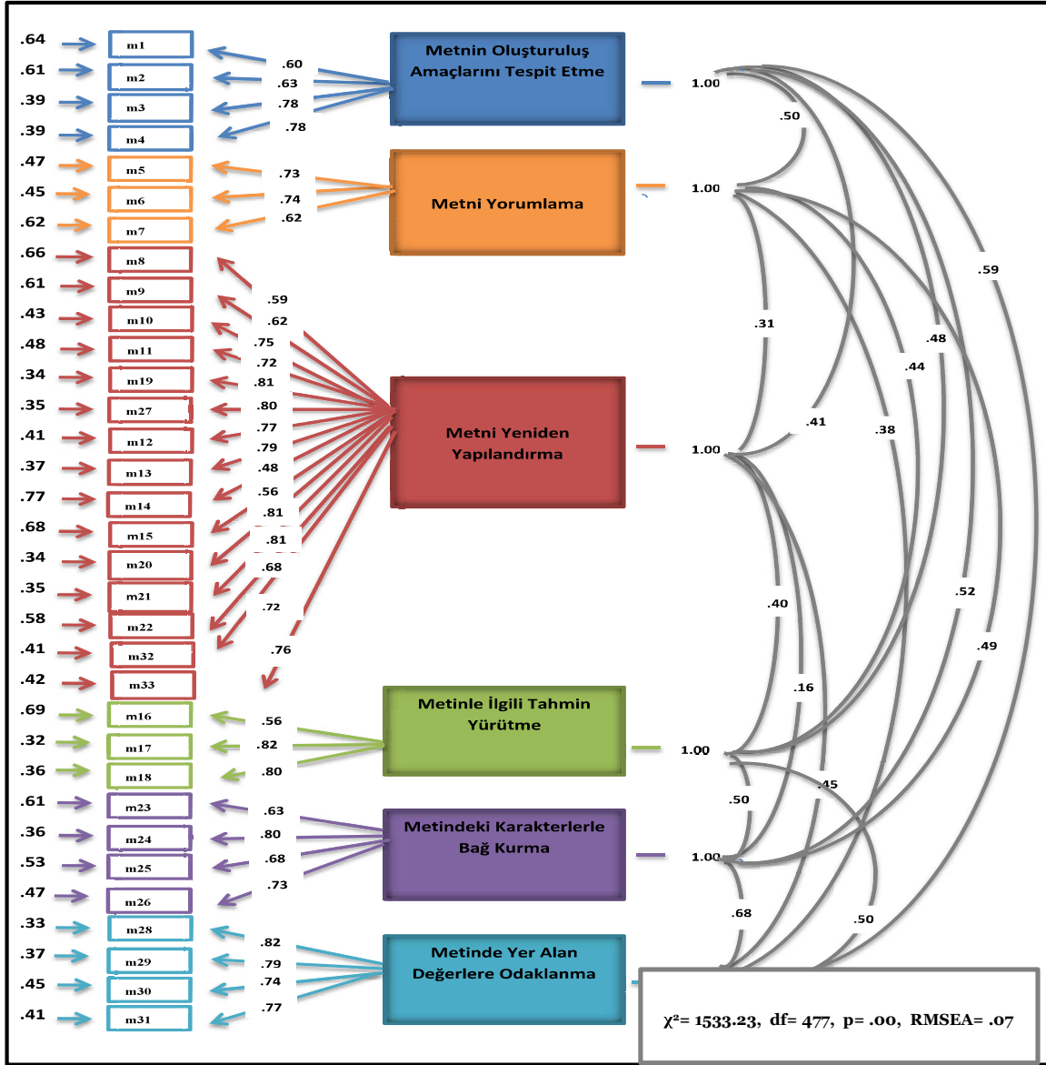
Şekil 2. YOBÖ'yü oluşturan faktörler arasındaki ilişki modeli
