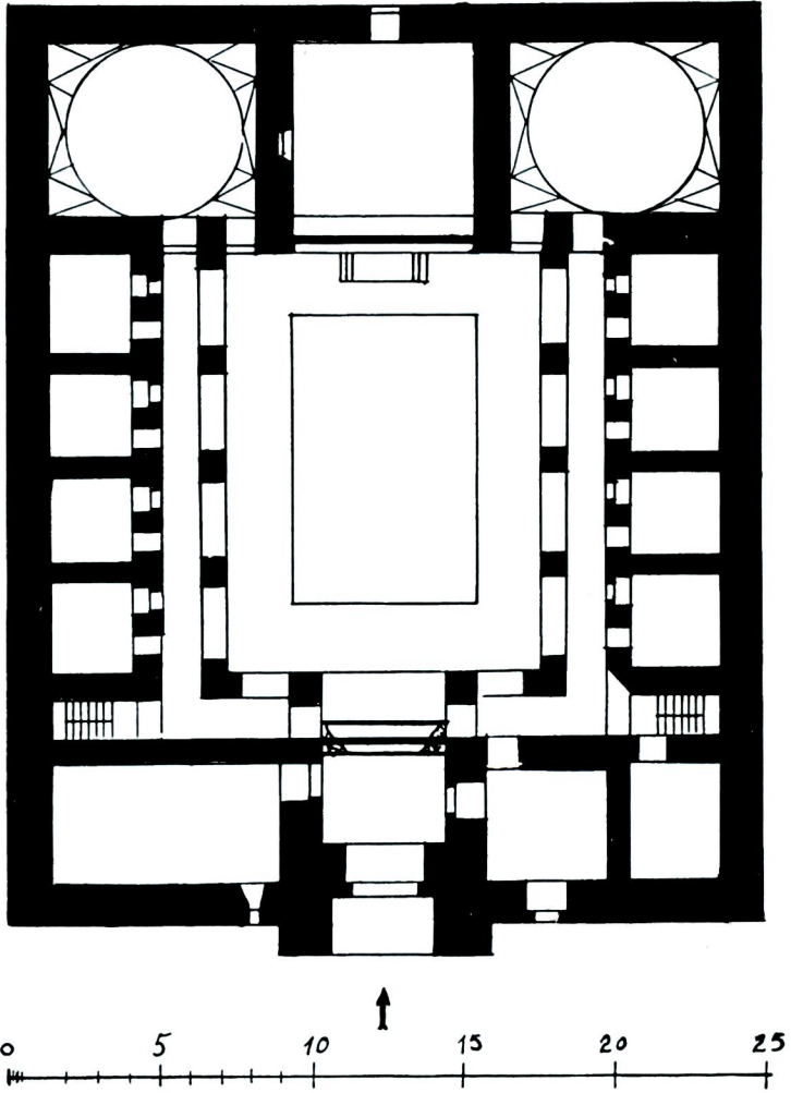
Plân. I — Sirça medrese pîlânı (Friedrich Sarre. Anadolu'da Seyyahat)a göre.
