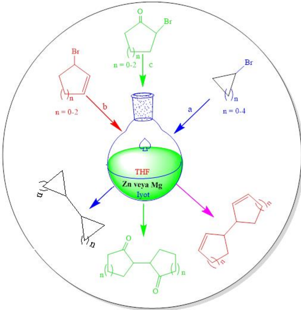
Şema 2. Kenetlenme Reaksiyonlarının Genel Şeması
