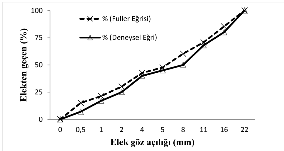
Şekil 2. Agrega granülometrisi
