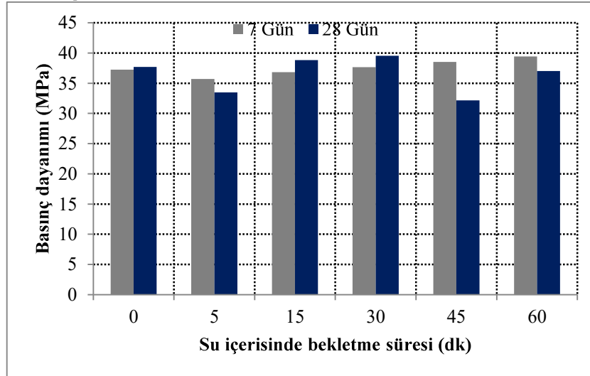
Şekil 7: Su içerisinde bekletme süresinin basınç dayanımı üzerindeki etkisi
