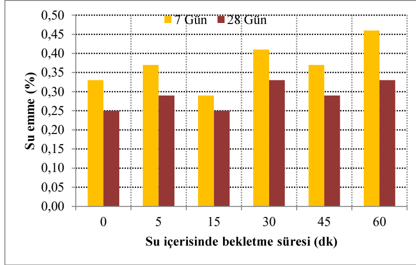
Şekil 6: Su içerisinde bekletme süresinin su emme üzerindeki etkisi
