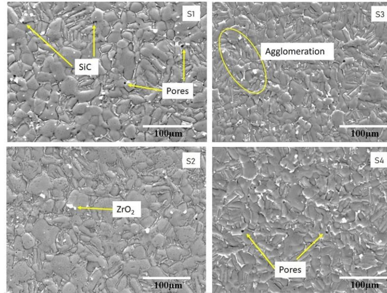
Figure 7. SEM Images of, (S1). Al – 5w/w.% SiC, (S2). Al – 5w/w.% SiC – 5w/w.% ZrO 2 , (S3). Al – 5w/w.% SiC – 10w/w.% ZrO 2 , (S4). Al – 5w/w.% SiC – 15w/w.% ZrO 2
