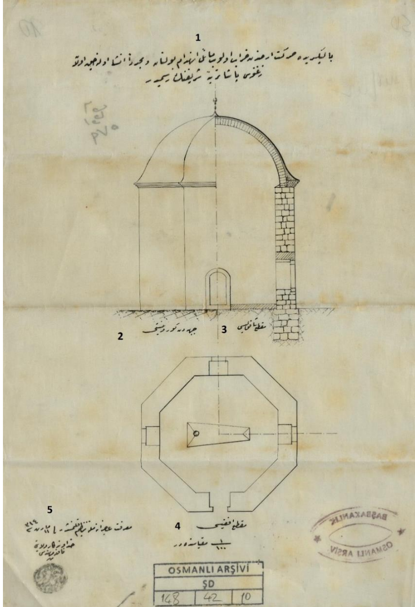
Görsel 8. Türbeye ait ilk çizim. 1. Balıkesir’de hareket-i arzdan harâb olub mâil-i inhidâm bulunan ve müceddeden inşâ olunacak olan Zağanos Paşa türbe-i şerîfinin resmidir. 2. Cepheden görünüşü. 3. Makta’-ı şâkûlîsi. 4. Makta’-ı ufkîsi 1/100 mikyâsındadır. 5. Ma’rifet-i ‘âcizânemle tanzîm kılınmışdır fi 11 Mart sene 314. Hüdâvendigâr Vilâyeti Nâfi’a Mühendisi Ahmed Fevzi (BOA., ŞD., 148/42).
