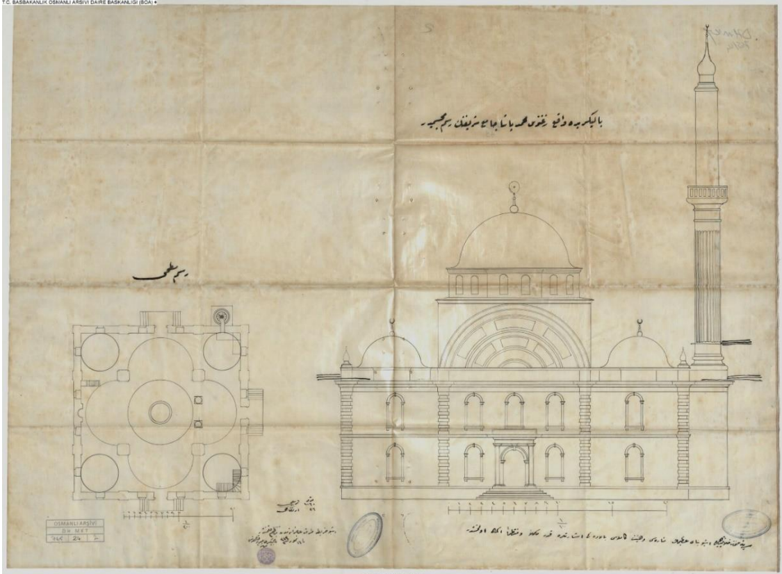
Görsel 5. Balıkesir belediye kalfası tarafından 16 Temmuz sene 1319/29 Temmuz 1903 tarihinde yapılan ikinci çizim. Caminin ön cephe görüntüsünün iki tarafına yapılan işaretler, inşaatın geldiği noktayı göstermektedir (BOA., DH.MKT., 765/24).
