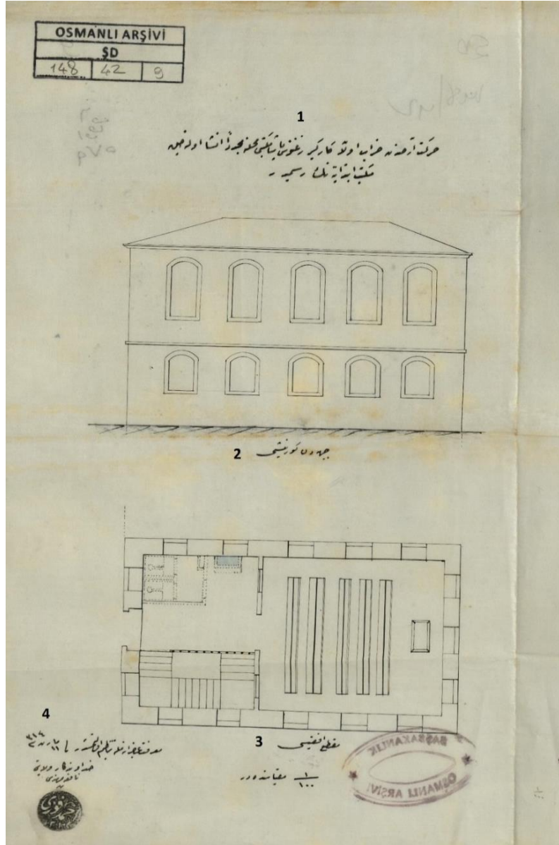
Görsel 10. 1. Hareket-i arzdan harâb olan kâgîr Zağanos Paşa mektebi mahalline müceddeden inşâ olunacak mekteb-i ibtidâiyenin resmidir. 2. Cepheden görünüşü, 3. Makta'-ı ufkîsi 1/100 mikyasındadır. 4. Ma'rifet-i 'âcizânemle tanzîm olunmuşdur fi 11 Mart sene 314. Hüdâvendigâr Vilâyeti Nâfi'a Mühendisi Ahmed Fevzi (BOA., ŞD., 148/42).
