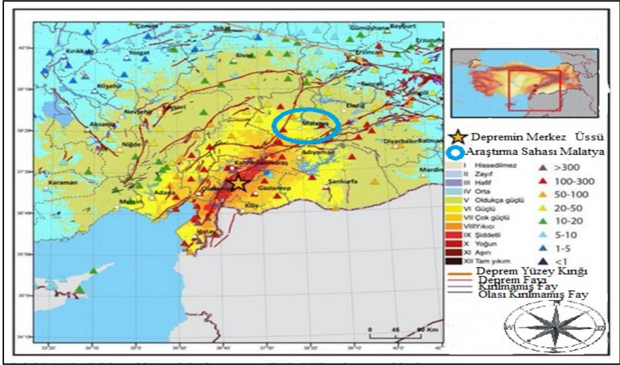
Harita 1. 6 Şubat 2023 Kahramanmaraş Merkezli Depremlerin Etki Alanları
