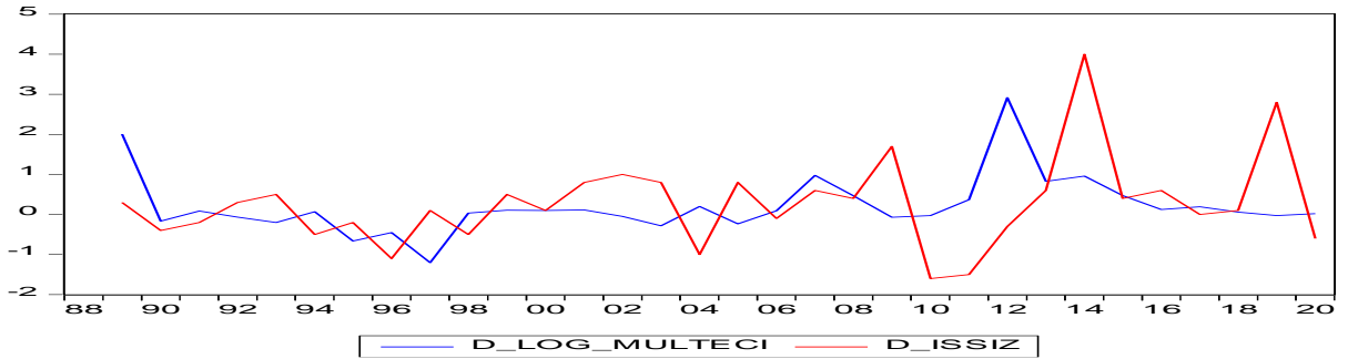
Şekil 1: Durağanlaştırılmış Serilere Ait Grafikler
