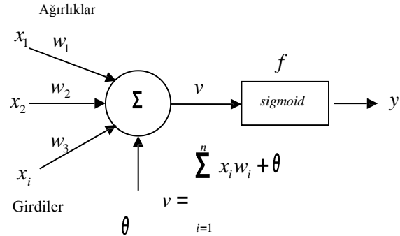
Şekil 1. Temel Yapay Sinir Ağı Hücresi: Yapay Nöron
