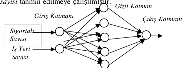
Şekil 3. Türkiye için YSA İş Kazası Modeline ait Ağ Mimarisi
