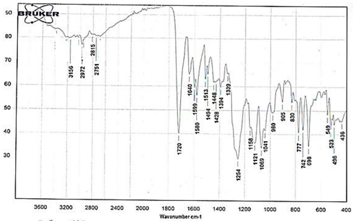
IR SPECTRUM OF L2-Fe
