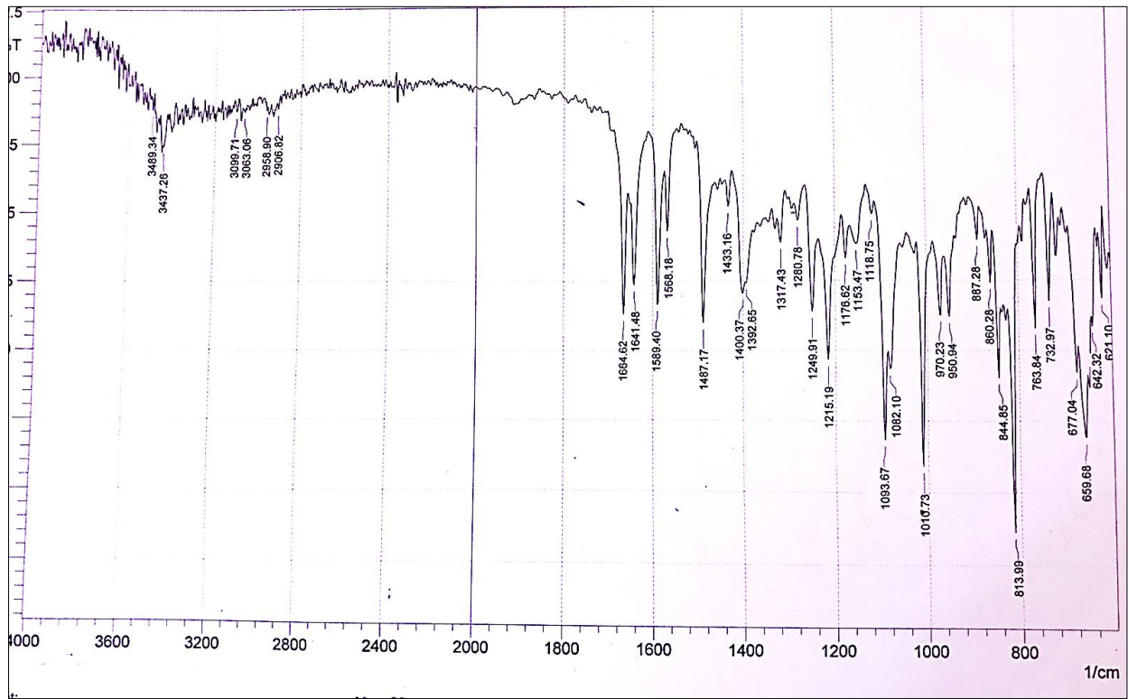
IR spectrum of L1-Fe
