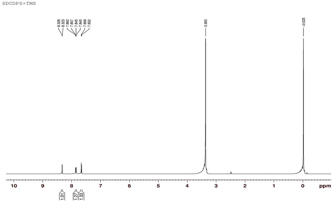
Şekil 2. S-DCDPS monomerin ^1\text{H} NMR spektrumu
