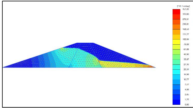
Şekil 10. Barajlarda oluşan sızmaya örnek (Example for seepage through dams)
