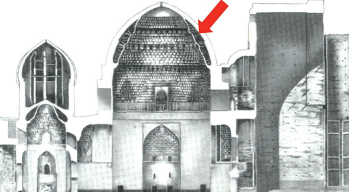
Şekil 3: XV. yüzyılın başında inşa edilen Hoca Ahmet Yesevi türbesinin çizimi. Kazanlık kubbесinin iç yapısı. Bu oyukta desenli ahşaplar bulunmuştur.
