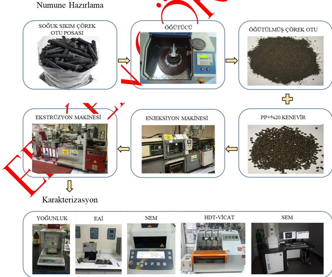
Şekil 2. PP+%20 kenevir/çörek otu/MAPP polimer kompozitinin üretim aşamaları ve kullanılan cihazlar (Production stages of PP+20% hemp/black cumin/MAPP polymer composite and devices used)
