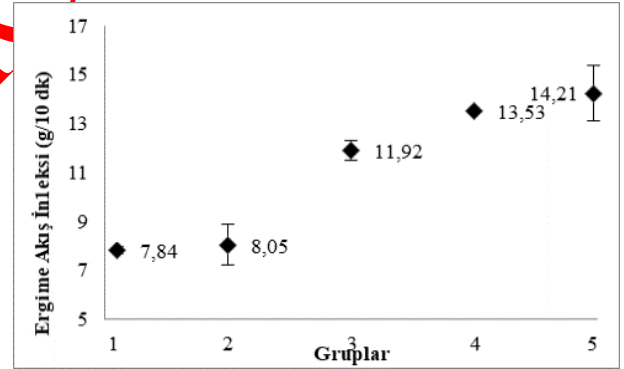
Şekil 4. PP+%20 kenevir/çörek otu/MAPP polimer kompozitinin EAİ değerleri (MFI values of PP+20% hemp/black cumin/MAPP polymer composite)
