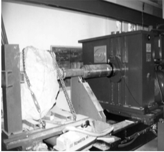
Şekil 2. Yatay sondaj makinesi.
