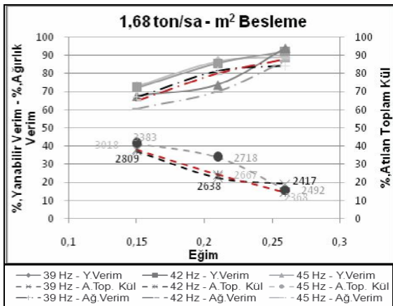
Şekil 16. Tabla eğimi – yanabilir verim, atılan toplam kül oranı (1,68 ton/saat - m 2 ).
