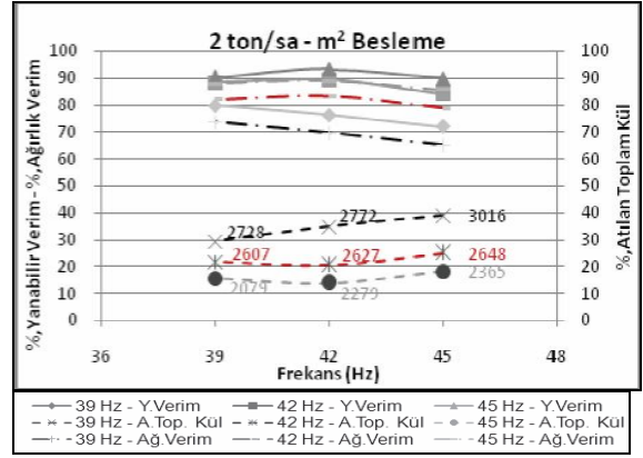
Şekil 18. Tabla frekansı – yanabilir verim, toplam atılan kül oranı (2 ton/saat - m 2 ).
