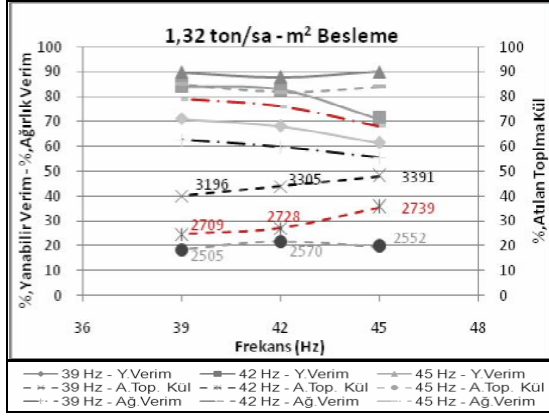
Şekil 20. Tabla frekansı - yanabilir verim, toplam atılan kül oranı (1,32 ton/saat - m 2 )
