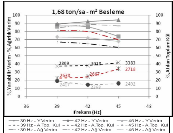
Şekil 19. Tabla frekansı – yanabilir verim, toplam atılan kül oranı (1,68 ton/saat - m 2 ).
