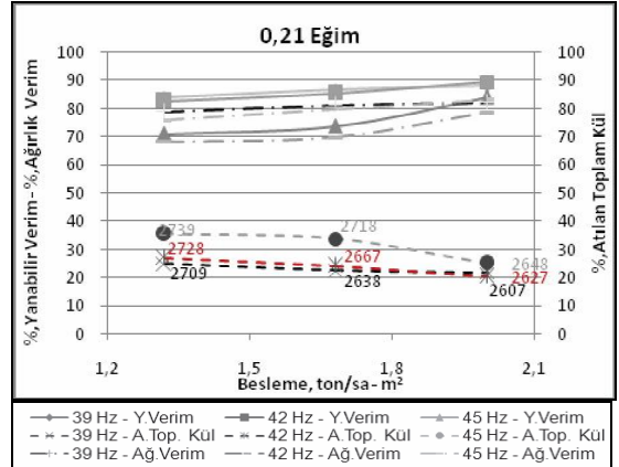
Şekil 13. Besleme – yanabilir verim, ağırlık verim, atılan top kül oranı (0,21 Eğim).
