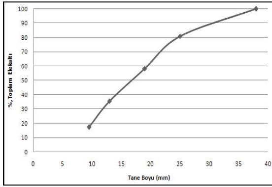
Şekil 8. Soma-Eynez numunesi tane boyu dağılımı.
