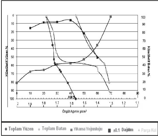
Şekil 9. Yeniköy-Hisarönü numunesi yıkanabilirlik eğrileri.
