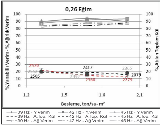
Şekil 14. Besleme – yanabilir verim, ağırlık verim, atılan top kül oranı (0,26 Eğim).
