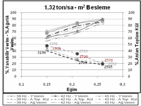
Şekil 17. Tabla eğimi – yanabilir verim, atılan toplam kül oranı (1,32 ton/saat - m 2 ).
