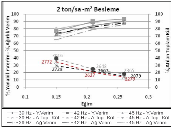
Şekil 15. Tabla eğimi – yanabilir verim, atılan toplam kül oranı (2 ton/saat - m 2 ).
