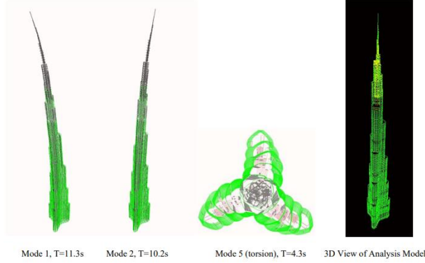
Şekil 33. Üç Boyutlu Analiz Modeli ve Dinamik Mod Şekilleri [5].
