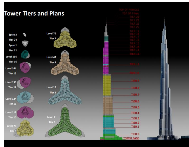
Şekil 5. Kulenin katman ve planları [27].
