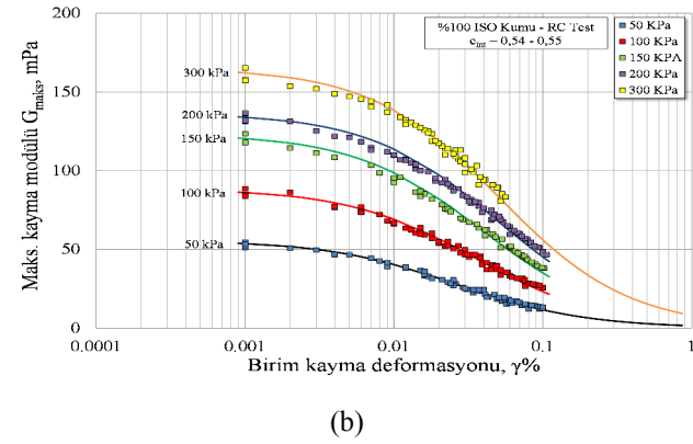
Şekil 4. %100 ISO temiz kuma ait (a) sönüm oranı, (b) maksimum kayma modülü verileri ve eğilim çizgileri
