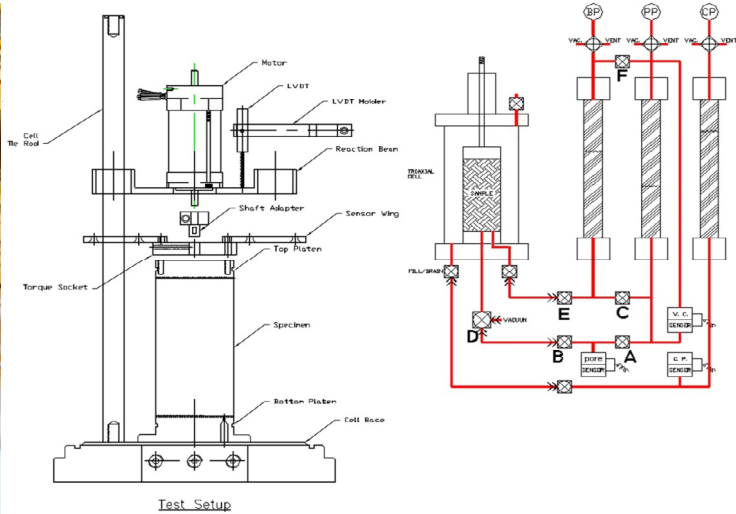
Şekil 1. Deneylerde kullanılan test sistemi ve en kesiti
