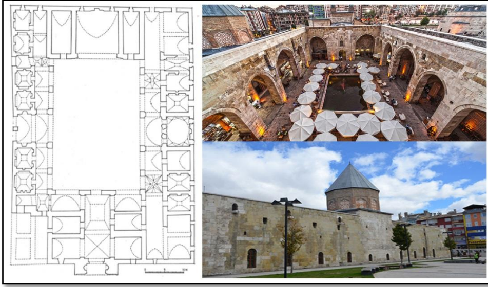
Resim 20. İzzeddin Keykâvus Dârüşşifâsı (Şifâiye Medresesi) Planı ve Eyvanları
