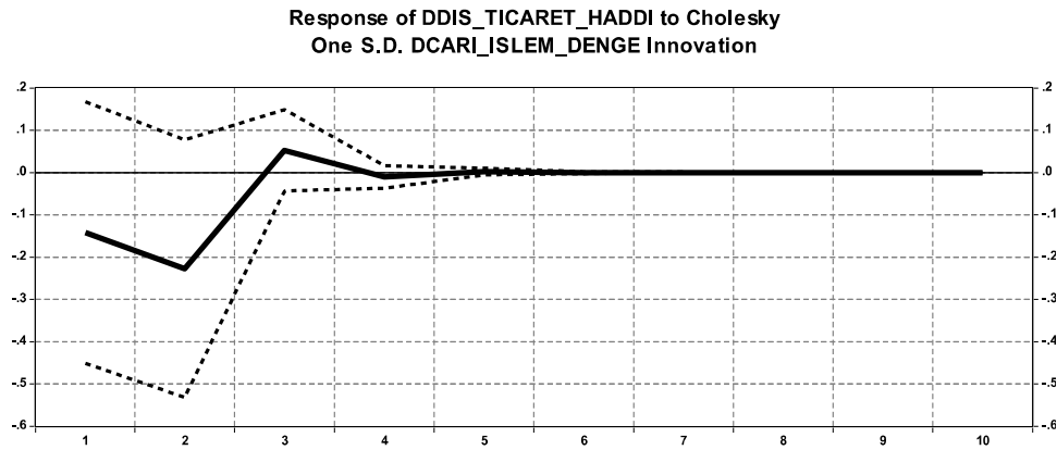
Şekil 4. Değişkenler İçin Etki-Tepki Grafikleri
