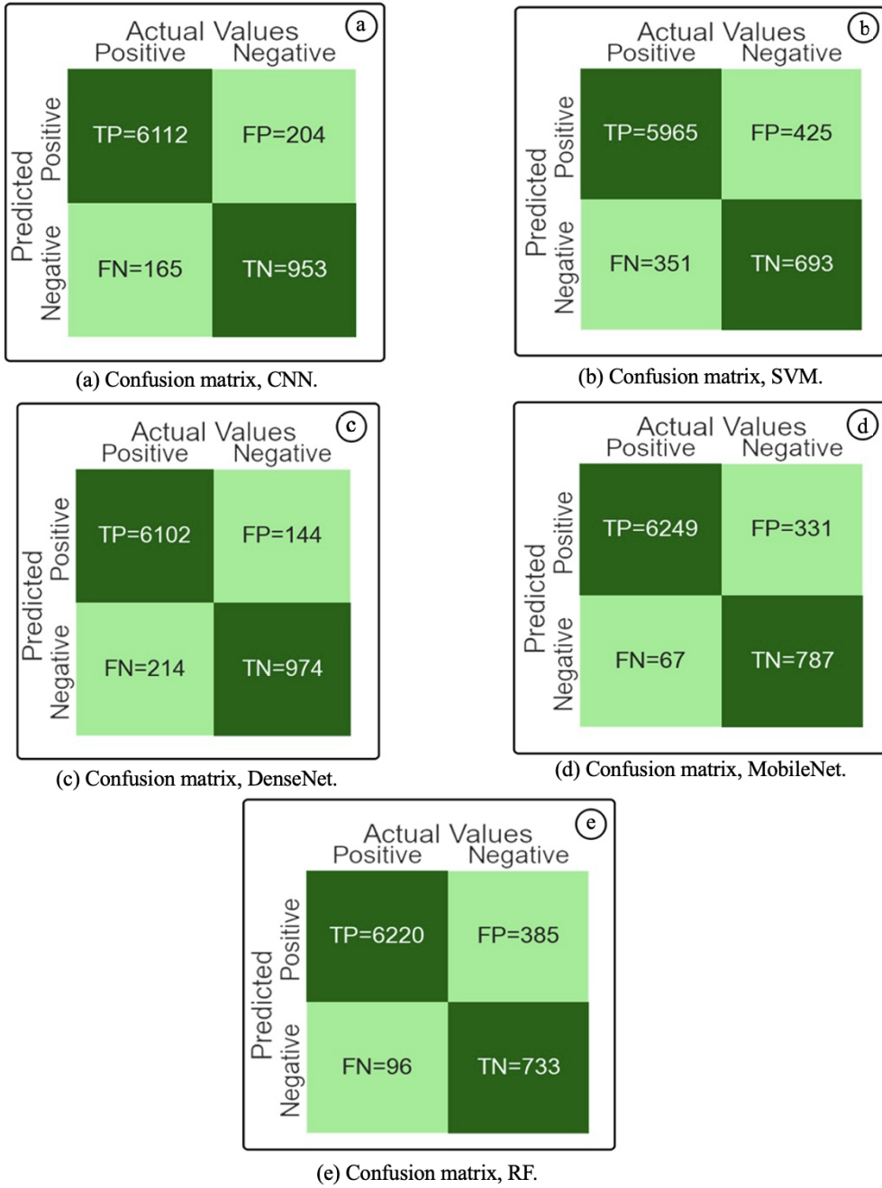
Figure 8. (a) CNN, (b) SVM, (c) DenseNet, (d) MobileNet, (e) RF Confusion matrices.
