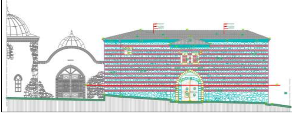
Şekil 20: Restore Edilen Yapının Güney Cephesi 78
