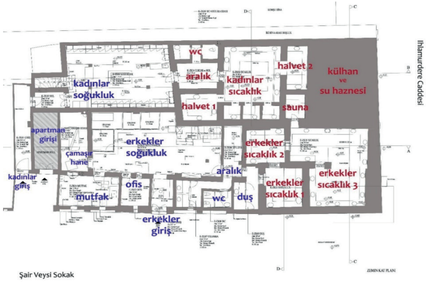
Şekil 3. Zemin kat planı - rölöve
