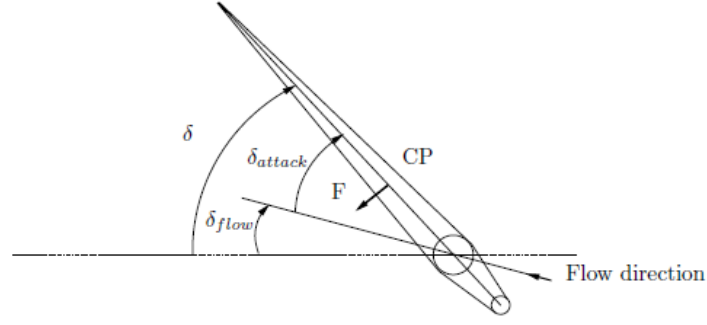
Şekil 1. Dümen açıları (SNAME, 1950).
