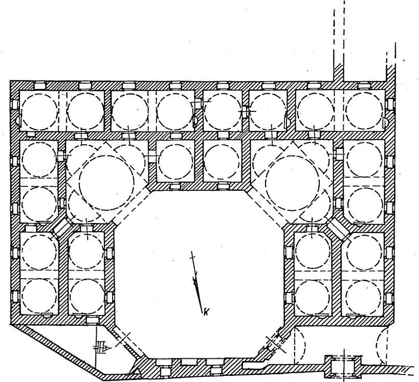
Plan 2: Haseki Darüşşifası planı.
