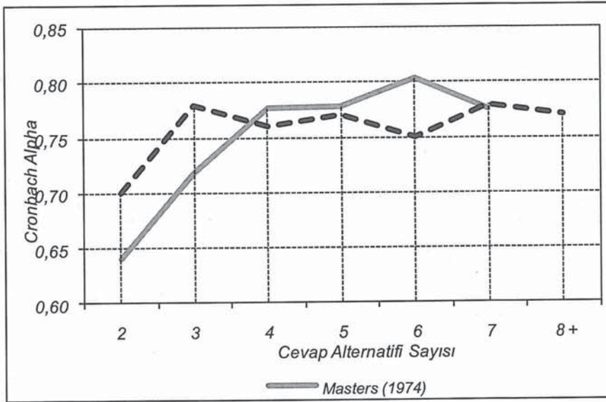
Şekil 1: Cevap Alternatifi Sayısı İle Cronbach Alpha Arasındaki İlişki
