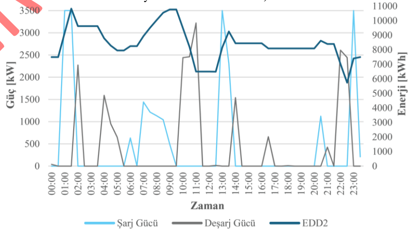
Şekil 11. Durum 1’de Bara 5’teki ED sisteminde güç ve enerji değerleri (Power and energy values of the ES system at Bus 5 in Case 1)
