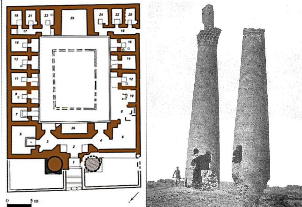
Plân 5) Medrese plânı (Smagulov 2016'dan düzenlenerek aktarılmıştır). Fotoğraf 9) Medresenin günümüze ulaşamayan minareleri (Baitanayev 2013).
