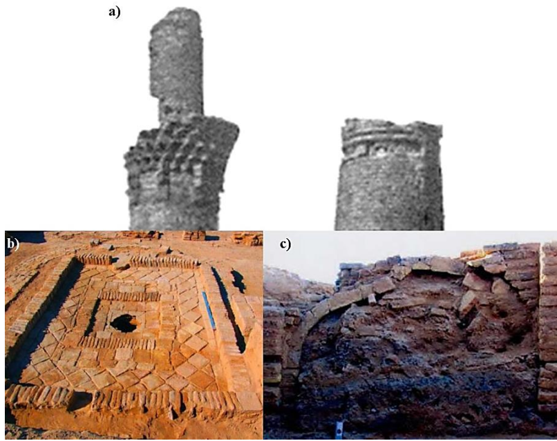
Fotoğraf 12 a) Minarelerdeki tuğla işçiliği. b) Cami abdesthane zemin düzenlemesi. c) Hankâh kaş kemer düzenlemesi.
