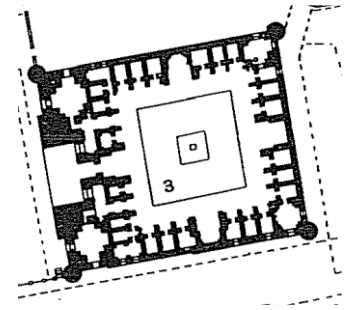
Şir-Dar Medresesi Plânı (Cezar 1977).
