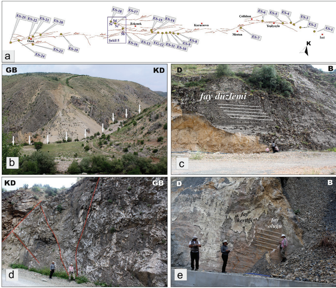
Şekil 5. Erkenek Segmenti'nin Karanlık Dere boyunca morfolojik gözlemleri: a) Erkenek segmenti boyunca gerçekleştirilen arazi çalışmalarına ait lokasyonların şematik harita üzerinde görünümü, b) Erkenek Segmenti'nin denetlediği vadi, c) Erkenek Segmenti'ne ait fay düzleminin görünümü, d) yoğun deformasyon sonucu gelişmiş makaslama kırıklarının mostra görünümü, e) kinematik göstergelerin net bir şekilde gözlemlendiği fay düzlemi.
