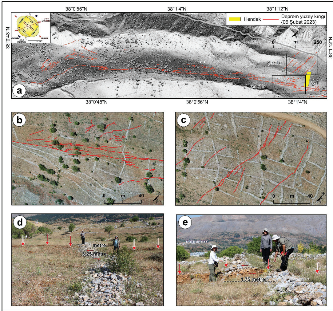
Şekil 7. Çelikhana güneyinde haritalanan 6 Şubat 2023 deprem yüzey kırığı üzerindeki deformasyonlar. a) Haritalanan yüzey kırığının yüksek çözünürlüklü SYM görüntüsü, b, c) Haritalanan yüzey kırığının yüksek çözünürlüklü ortofoto üzerinde görünümü, d, e) Cilke sırtında gözlemlenen sol yanal yer değiştirmeler (d: 38.018722° K, 38.239794° D; e: 38.020319° K, 38.239989° D). Bakış yönü sırasıyla kuzey) ve kuzeybatıdır.
