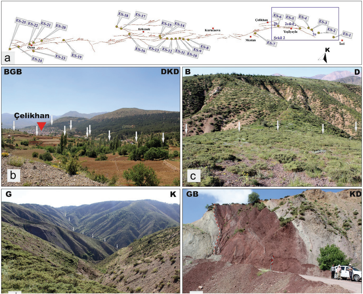
Şekil 2. Erkenek segmentinin kuzeydoğu ucundaki morfolojik gözlemler: a) Erkenek segmenti boyunca gerçekleştirilen arazi çalışmalarına ait lokasyonların şematik harita üzerinde görünümü, b) Çelikhan yerleşim yerinin kuzey ve güney kenarını sınırlayan Erkenek segmentinin arazi görünümü, c) Yeşilyayla civarında Erkenek segmenti tarafından denetlenen boyunun arazi görünümü, d) boyunun devamında sağa doğru büküm yapan segmentin vadi boyunca görünümü, e) İzci'nin batısında iki farklı birim arasındaki tektonik dokanağı oluşturan Erkenek Segmenti'nin mostra görünümü.
