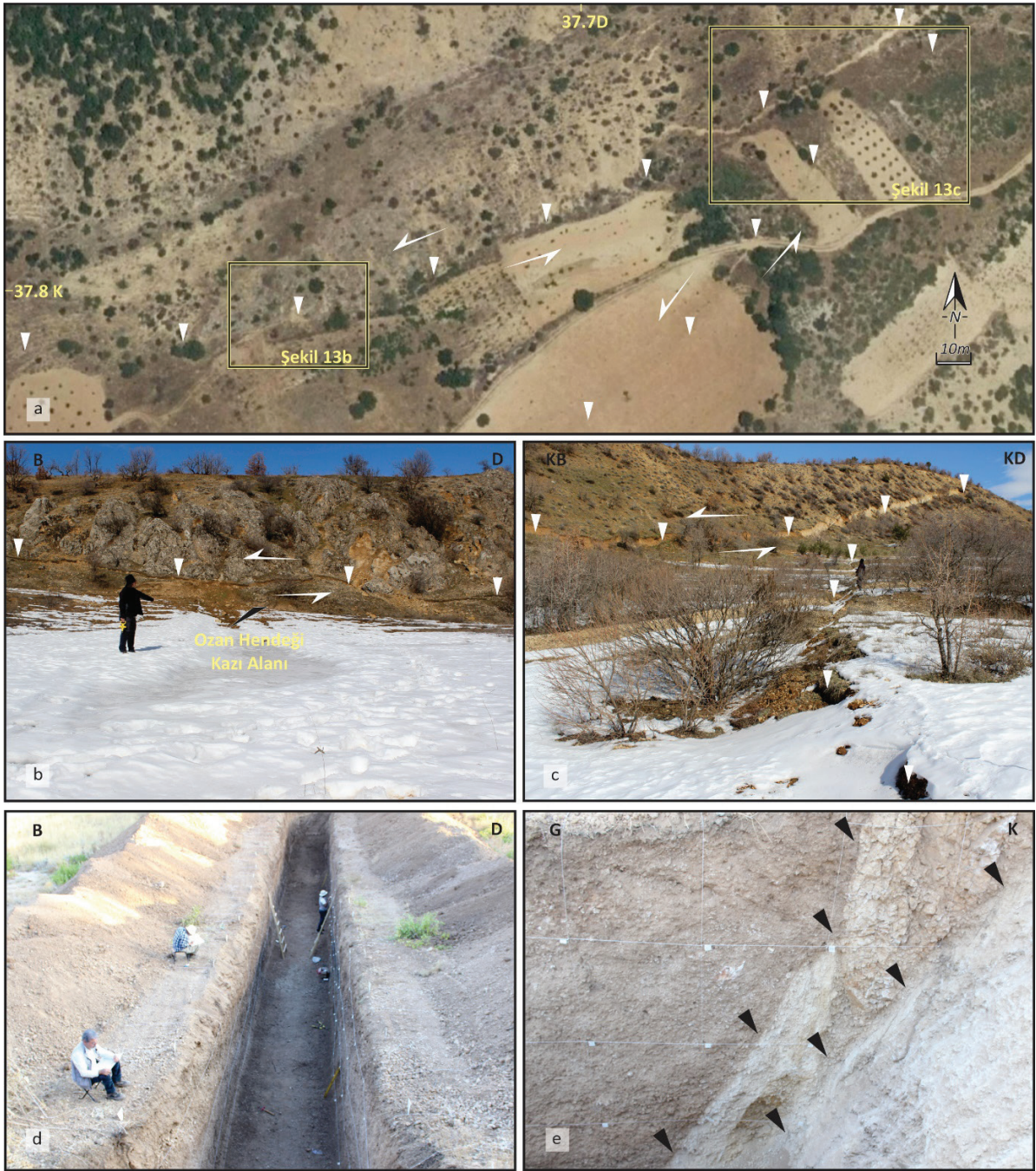
Şekil 13. a) DAFZ Erkenek segmenti üzerinde açılmış olan Ozan hendeğinin 6 Şubat 2023 tarihli depremler sırasında oluşmuş yüzey kırığına (beyaz üçgenlerle işaretlenmiş) göre konumu, b) hendek kazı alanının yüzey kırığı ile birlikte arazi görünümü, c) yüzey kırığının arazi görünümü, d) hendek çalışmaları, e) fayın hendek içi görünümü (siyah üçgenlerle işaretlenmiş).
