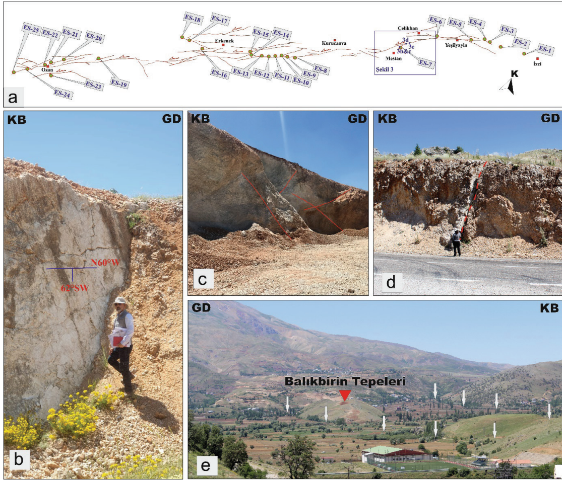
Şekil 3. Erkenek Segmentinin Çelikhan'daki morfolojik gözlemleri: a) Erkenek segmenti boyunca gerçekleştirilen arazi çalışmalarına ait lokasyonların şematik harita üzerinde görünümü, b) Çelikhan civarında Erkenek Segmenti'ne ait fay düzleminin görünümü, c) Erkenek Segmenti tarafından yoğun deformasyona uğramış ana deformasyon zonunun mostra görünümü, d) Kataklastik yapı kazanmış birimlerin faylanmış mostra görünümü, e) Erkenek Segmenti'nin ana deformasyon zonunda segmente paralel gelişmiş basınç sırtının arazi görünümü.
