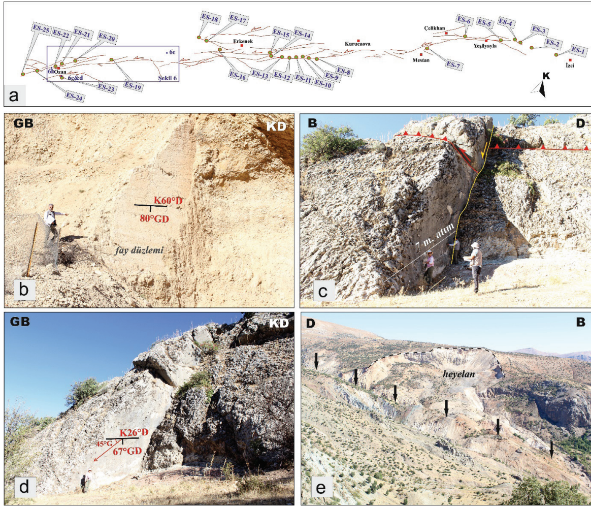
Şekil 6. Erkenek Segmenti'nin güneybatı ucundaki morfolojik gözlemler: a) Erkenek segmenti boyunca gerçekleştirilen arazi çalışmalarına ait lokasyonların şematik harita üzerinde görünümü, b) Erkenek Segmenti'nin fay düzleminin görünümü, c) Harmanlı mevkiinde Erkenek Segmenti tarafından yaklaşık 7 m sol yanal ötelenen önceki deformasyonların görünümü, d) Erkenek Segmenti fay düzleminin görünümü, e) büyük Akyar heyelanını kontrol eden Erkenek Segmenti'nin görünümü.
