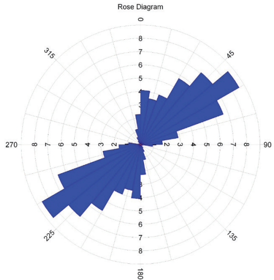
Şekil 8. Cilke sırtı boyunca ölçülen yüzey kırıklarından elde edilen doğrultu gül diyagramı.
