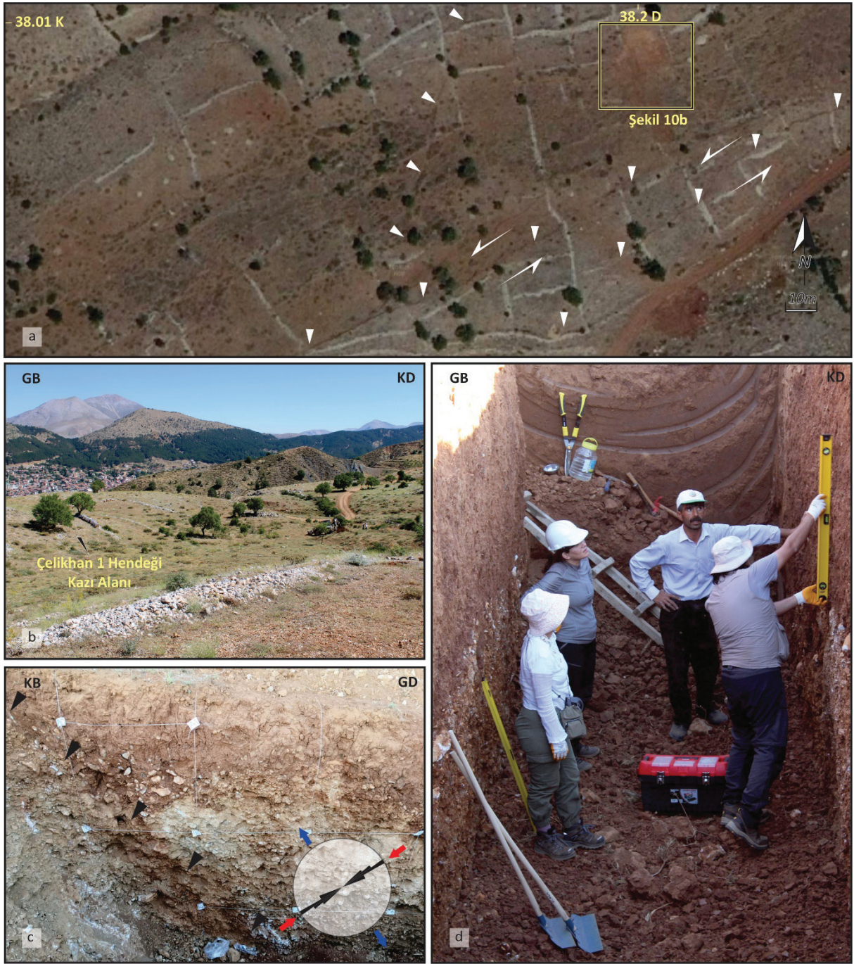
Şekil 10. a) DAFZ Erkenek segmenti üzerinde açılmış olan Çelikhan-1 hendeğinin 6 Şubat 2023 tarihli depremler sırasında oluşmuş yüzey kırığına göre (beyaz üçgenlerle işaretlenmiş) konumu, b) hendeğin kazı alanı arazi görünümü, c) doğrultu gül diyagramı ile fayın hendeğin içi görünümü (siyah üçgenlerle işaretlenmiş), d) hendeğin içi çalışmalar.
