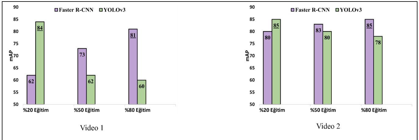
Şekil 12. Senaryo 2'de eğitime katılmadan sadece test için kullanılan her iki videonun mAP sonuçları.
