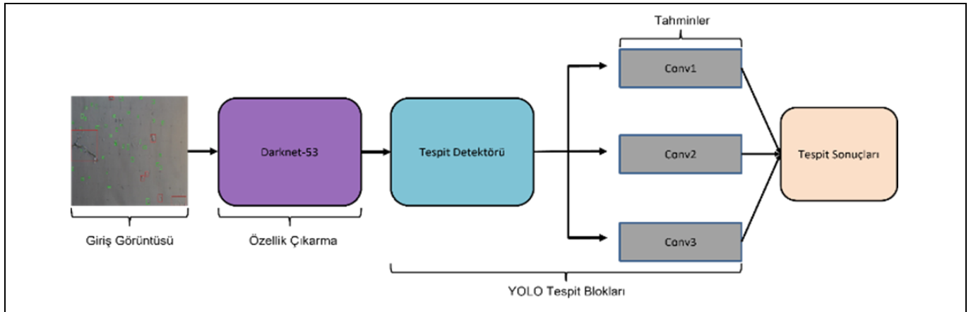
Şekil 6. YOLOv3 yönteminin genel yapısı [30].
