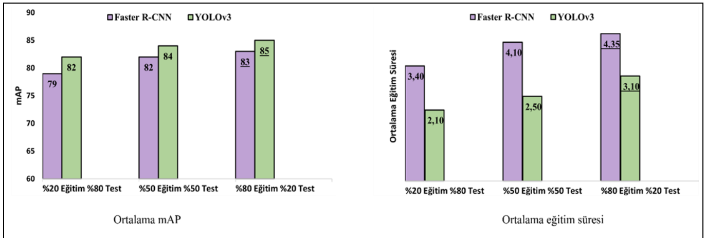
Şekil 11. Senaryo 1 için sekiz videonun ortalama mAP ve eğitim süresi sonuçları.
