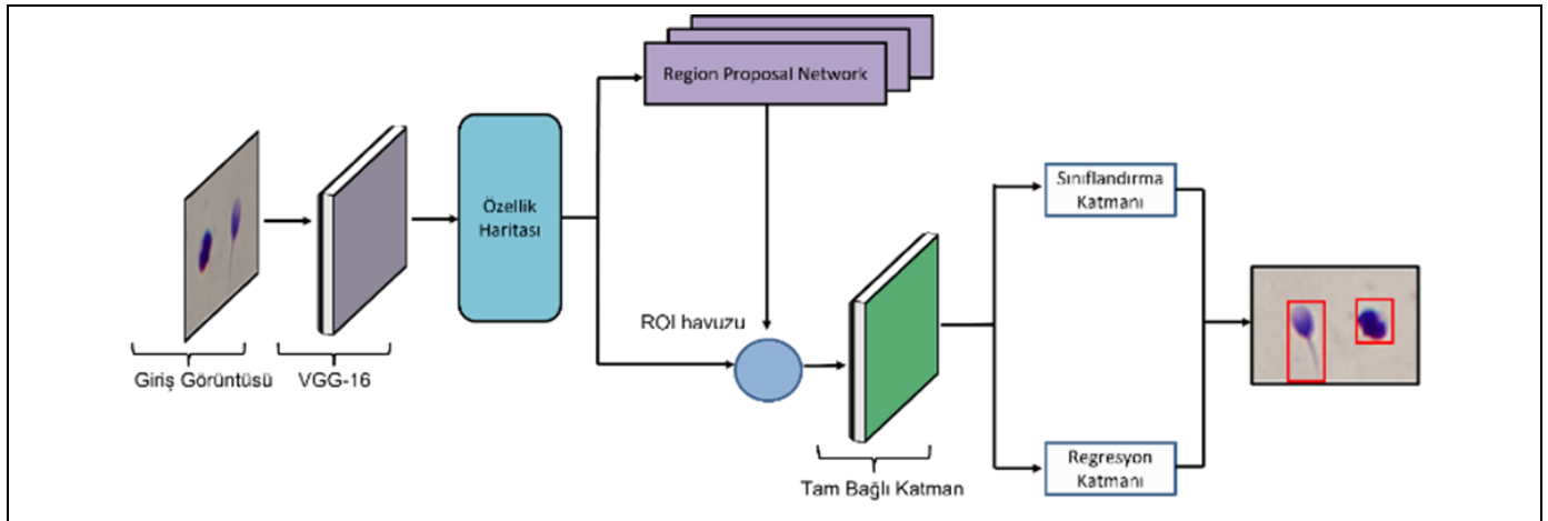
Şekil 7. Faster R-CNN modelinin genel yapısı [26].
