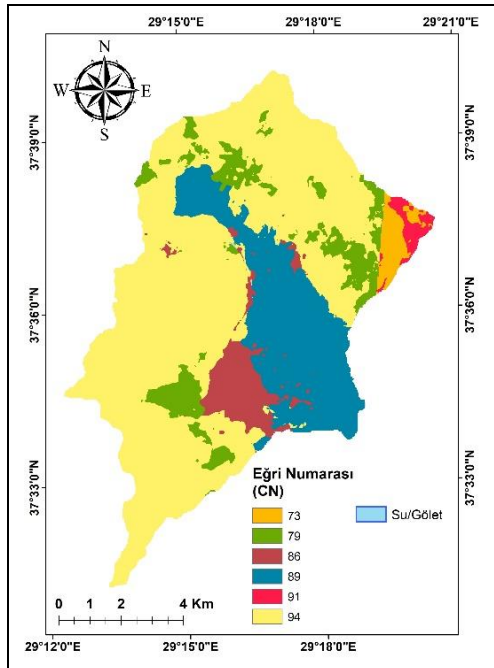
Şekil 5. Eğri numarası haritası.
