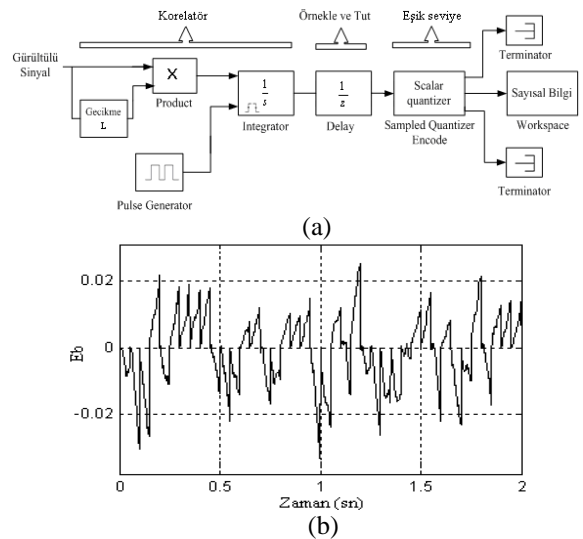
Şekil 5. KGKA demodülör (a) Simulink modeli (b) Korelatör çıkışı
