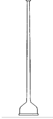
Çizim 2. Salpinks.
